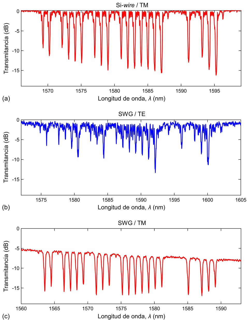
Figura 3.31. Respuesta en transmitancia medida para los filtros astrofotónicos, con las configuraciones de filtro: (a) Si-wire/TM, (b) SWG/TE y (c) SWG/TM. Las pérdidas del sistema de medida, de los edge-couplers y de las guías de interconexión han sido descontadas de las curvas mostradas.
