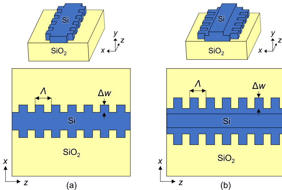
Figura 3.2. Representación esquemática 2D (vista superior) de filtros Bragg en tecnología SOI basados en guías con corrugaciones laterales, mediante (a) guía Si-wire y (b) guía rib . Para clarificar las diferencias entre ambas, se incluye una pequeña representación esquemática 3D en la parte superior.
