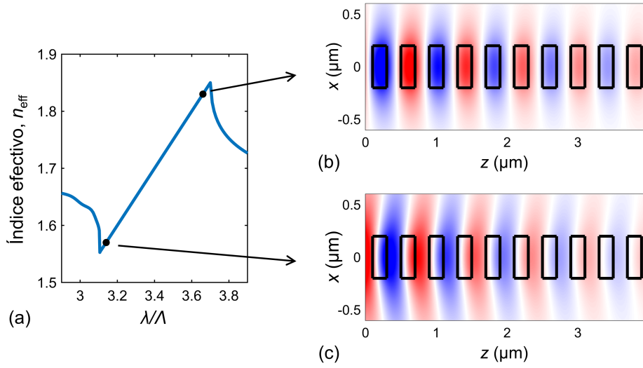
Figura 2.5. (a) Variación del índice efectivo Floquet-Bloch con respecto al cociente entre la longitud de onda y el periodo en torno a la primera zona de Bragg. Propagación de campo eléctrico (polarización TE) del modo Floquet-Bloch para diferentes puntos del bandgap , con (b) alto índice efectivo y (c) bajo índice efectivo. Los datos corresponden a la misma estructura que se ha analizado en las figuras 2.3 y 2.4. Simulación realizada para: (b) \lambda/\Lambda = 3.66 , y (c) \lambda/\Lambda = 3.14 .
