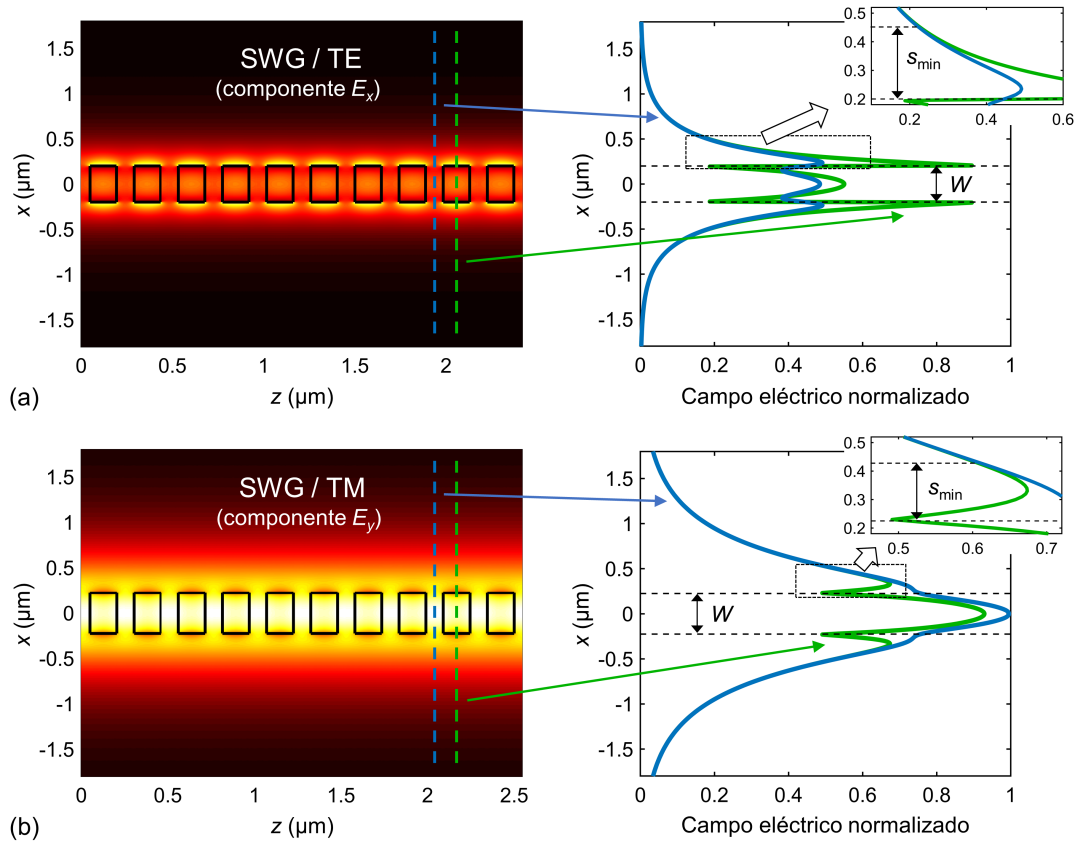
Figura 3.8. Propagación de la componente principal de campo eléctrico (módulo) del modo Floquet-Bloch de la guía SWG a lo largo de diez periodos, para los diseños con polarización (a) TE y (b) TM. A la derecha se representan los cortes transversales de campo en el centro del segmento de silicio (verde) y en el centro de la sección con dióxido de silicio (azul), incluyendo una ampliación de la zona donde ambos cortes comienzan a parecerse
