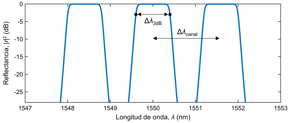
Figura 3.14. Reflectancia espectral objetivo de un filtro flat-top con tres canales en torno a la longitud de onda de 1550 nm.
