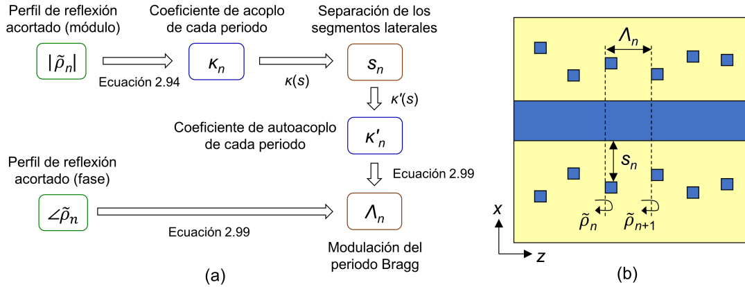
Figura 2.21. Representación gráfica del proceso de diseño de filtros Bragg apodizados con perturbaciones del campo evanescente propuesto en esta tesis. (a) Flujograma de los pasos a seguir para obtener los parámetros geométricos del filtro apodizado: las separaciones s_n y la longitud de cada periodo Bragg \Lambda_n . (b) Representación esquemática 2D (vista superior) de la estructura a diseñar.
