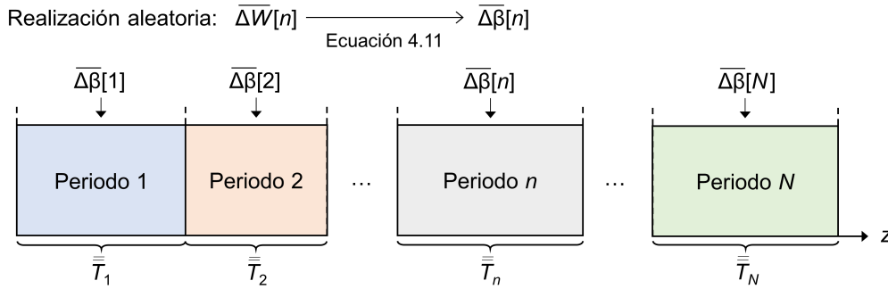
Figura 4.5. Representación esquemática del proceso de simulación de filtros con ruido de fase mediante el TMM, con (a) modelo de ruido de fase continuo, y (b) modelo de ruido de fase discreto.
