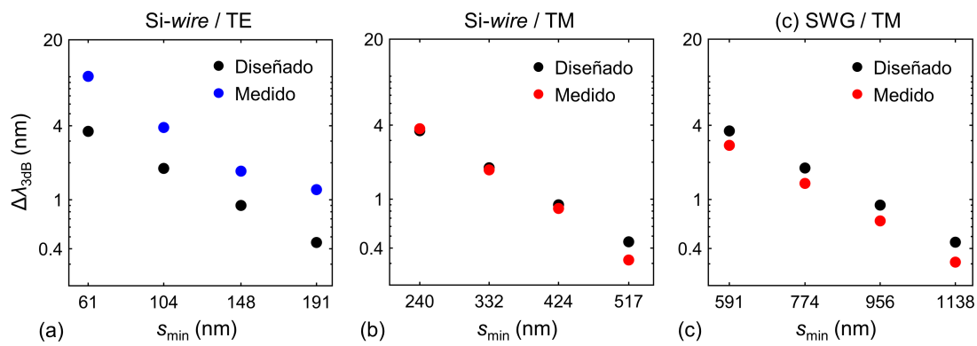
Figura 3.30. Comparación del ancho de banda a 3 dB diseñado y medido para los filtros sinusoidales, con las configuraciones de filtro: (a) Si-wire/TE, (b) Si-wire/TM y (c) SWG/TM. En el eje de abcisas se representa la separación mínima de los segmentos laterales correspondiente a cada diseño. Nótese que el eje vertical se representa en escala logarítmica (esto da lugar a una variación de tipo lineal del ancho de banda con respecto a la separación mínima de los segmentos).
