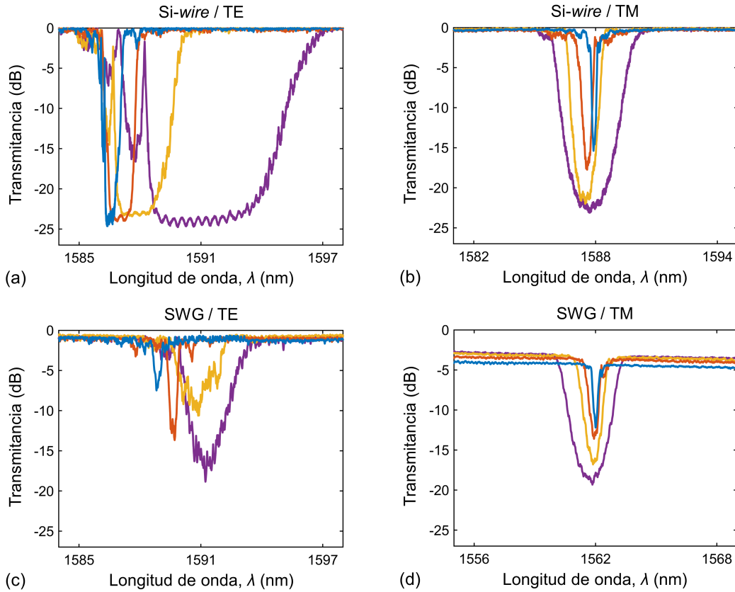
Figura 3.29. Respuesta en transmitancia medida para los filtros sinusoidales, con las configuraciones de filtro: (a) Si-wire/TE, (b) Si-wire/TM, (c) SWG/TE y (d) SWG/TM. En cada gráfica, cada curva representa una implementación de filtro distinta, con los siguientes anchos de banda nominales: \Delta\lambda_{3dB} = 0.45 nm (azul), \Delta\lambda_{3dB} = 0.90 nm (rojo), \Delta\lambda_{3dB} = 1.80 nm (amarillo), y \Delta\lambda_{3dB} = 3.60 nm (morado). Todos los diseños presentan un ER nominal de 25 dB. Las pérdidas del sistema de medida, de los edge-couplers y de las guías de interconexión han sido descontadas de las curvas mostradas.
