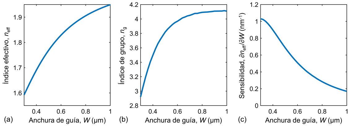
Figura 4.15. (a) Índice efectivo, (b) índice de grupo, y (c) sensibilidad del índice efectivo con la anchura de la guía, para el modo TM fundamental de una guía Si-wire y diferentes valores de anchura de la guía. Longitud de onda de operación: \lambda_0 = 1.55 \text{ nm} . Este resultado se ha obtenido mediante simulación electromagnética de la guía Si-wire (análisis modal).
