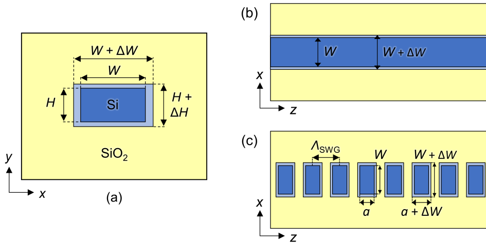
Figura 3.33. Representación esquemática de los errores de fabricación considerados para explicar el desplazamiento de la respuesta en los filtros fabricados: (a) vista frontal; (b) vista superior para filtros con núcleo Si-wire; (c) vista superior para filtros con núcleo SWG. En azul oscuro se delimitan las zonas de silicio del diseño nominal y en azul claro las dimensiones realmente fabricadas (con \Delta H, \Delta W > 0 ).
