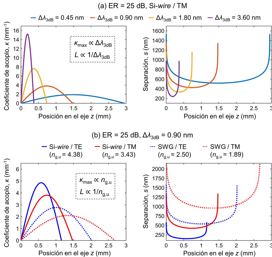
Figura 3.13. Comparativa de perfiles de coeficiente de acoplo y separación lateral de filtros sinusoidales, (a) para diferentes anchos de banda a 3 dB y (b) para diferentes configuraciones de filtro. En ambos casos, se especifica un ER objetivo de 25 dB. La comparativa (a) se realiza para la configuración de filtro basada en núcleo Si-wire y polarización TM. La comparativa (b) se realiza manteniendo un ancho de banda a 3 dB objetivo de 0.90 nm.
