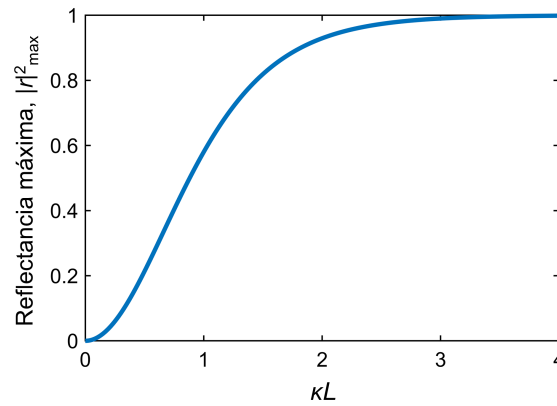
Figura 2.12. Variación de la reflectancia máxima de un filtro Bragg no apodizado en función del producto entre el coeficiente de acoplo y la longitud del filtro.
