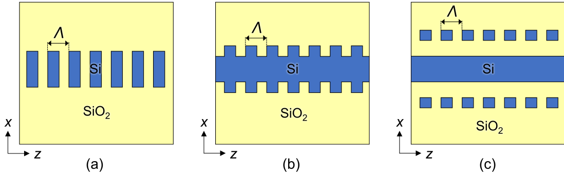
Figura 2.1. Representación esquemática 2D (vista superior) de algunas estructuras periódicas típicas en la plataforma SOI: (a) guía con núcleo segmentado; (b) guía con corrugaciones laterales; (c) guía con perturbación del campo evanescente.
