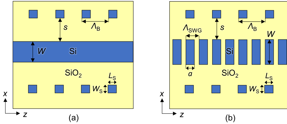
Figura 3.9. Representación esquemática 2D (vista superior) de las estructuras Bragg no apodizadas a analizar para determinar las funciones características de acoplamiento, \kappa(s) y \kappa'(s) , con (a) núcleo Si-wire y (b) núcleo SWG.
