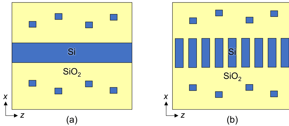
Figura 1.6. Representación esquemática 2D (vista superior) de las topologías de filtro Bragg apodizado propuestas y analizadas en esta tesis doctoral, con (a) guía Si-wire y (b) guía SWG.
