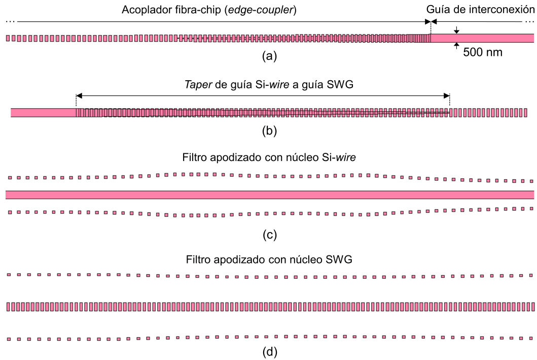
Figura 3.21. Capturas de diferentes zonas de la máscara definida para fabricar los filtros: (a) transición de acoplador fibra-chip a guía de interconexión de entrada; (b) taper de guía Si-wire a guía SWG; (c) sección del filtro astrofotónico con núcleo Si-wire para polarización TM; (d) sección del filtro astrofotónico con núcleo SWG para polarización TM.
