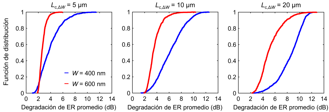
Figura 4.18. Análisis del impacto del ruido de fase en filtros astrofotónicos con diferentes anchuras de guía: funciones de distribución acumuladas correspondientes a la degradación del ER promedio de los 20 notches del filtro para diferentes longitudes de correlación L_{c,\Delta W} . Cada color identifica el diseño correspondiente a una anchura de guía, siendo todos los filtros diseñados para la configuración con núcleo Si-wire y polarización TM. Se han simulado un total de 1000 realizaciones aleatorias por caso, con una desviación típica \sigma_{\Delta W} = 2 nm.
