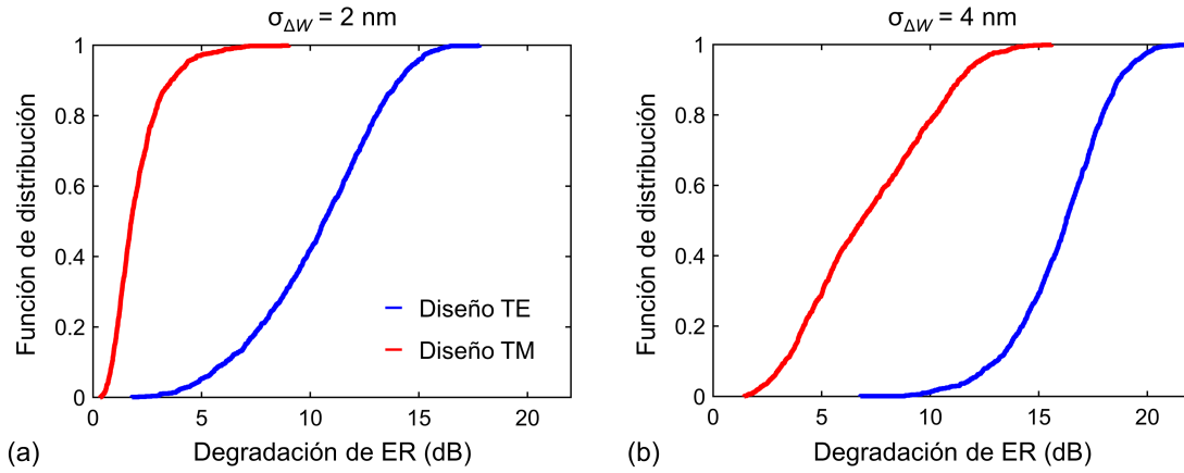
Figura 4.12. Análisis del impacto del ruido de fase en filtros sinusoidales con diferentes polarizaciones de trabajo: funciones de distribución acumuladas correspondientes a la degradación de ER para desviaciones típicas (a) \sigma_{\Delta W} = 2 nm y (b) \sigma_{\Delta W} = 4 nm. Cada color identifica el diseño correspondiente a una polarización, con ambos teniendo el mismo ER y ancho de banda nominales. Se han simulado un total de 1000 realizaciones aleatorias por caso, con una longitud de correlación L_{c,\Delta W} = 15 \mu\text{m} .
