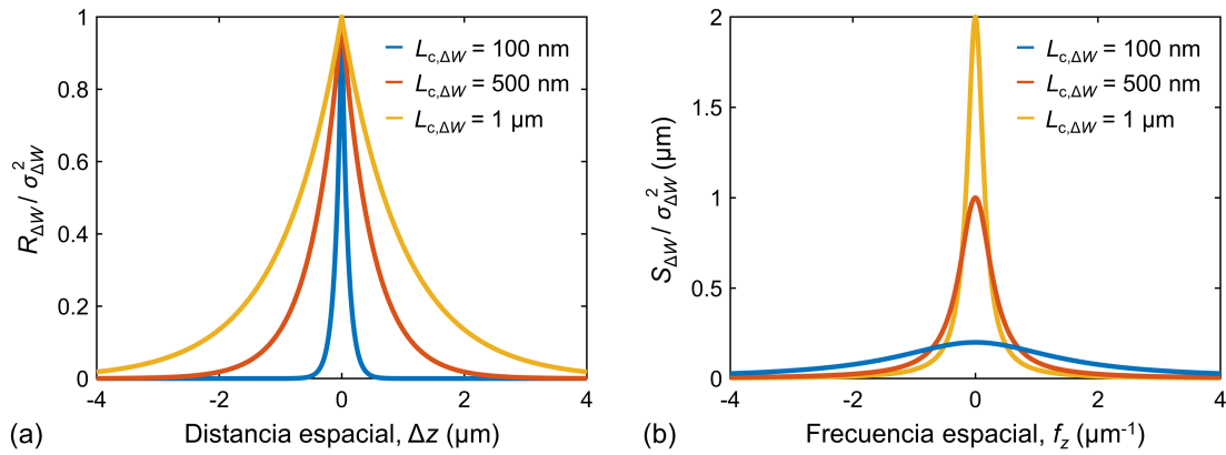
Figura 4.2. (a) Función de autocorrelación de \Delta W(z) en función de la distancia espacial \Delta z , y (b) densidad espectral de potencia de \Delta W(z) en función de la frecuencia espacial f_z , ambas normalizadas por la varianza del proceso \sigma_{\Delta W}^2 . Se proporcionan curvas para diferentes longitudes de correlación L_{c,\Delta W} : 100 nm (azul), 500 nm (rojo), y 1 \mu\text{m} (amarillo).
