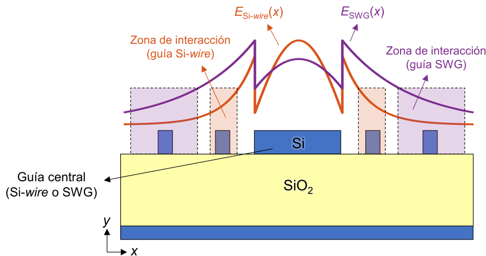
Figura 1.5. Representación esquemática 2D (vista frontal) de la interacción entre campo eléctrico y perturbaciones en filtros Bragg basados en perturbación del campo evanescente. Las curvas representan los perfiles de campo eléctrico de una guía Si-wire convencional (rojo) y de una guía SWG con bajo confinamiento modal (morado). Las regiones marcadas con líneas discontinuas comparan zonas con misma fuerza de interacción entre campo eléctrico y perturbaciones. El área de esta zona aumenta al reducir el confinamiento modal, permitiendo un control más preciso de las características del filtro. También se incrementa la fuerza de interacción para la mínima separación de las perturbaciones permitida en fabricación.
