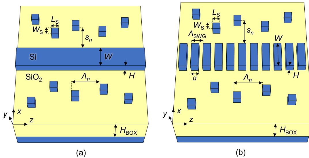
Figura 3.6. Representación esquemática 3D de las geometrías propuestas en esta tesis para diseñar filtros Bragg apodizados con respuestas espectrales arbitrarias en tecnología SOI, con (a) núcleo Si-wire y (b) núcleo SWG. La estructura comprende un sustrato de silicio, una capa de dióxido de silicio o BOX de altura H_{\text{BOX}} (típicamente 2 o 3 \mu\text{m} ), un núcleo de silicio de altura H = 220 nm, y un recubrimiento o cladding superior de dióxido de silicio (no mostrado en la figura por claridad).
