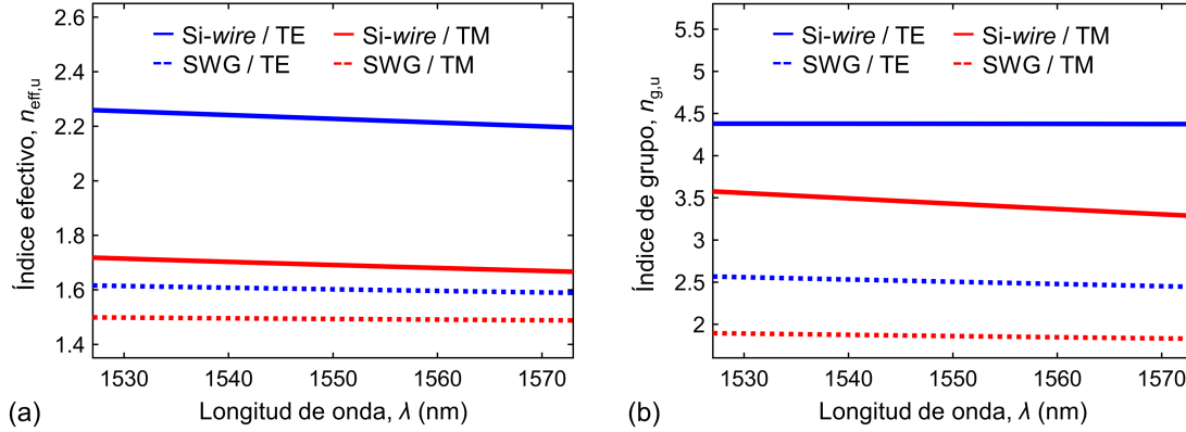
Figura 3.7. (a) Índice efectivo e (b) índice de grupo de la guía sin perturbar ( Si-wire o SWG) en función de la longitud de onda para las diferentes configuraciones estudiadas. Los parámetros geométricos utilizados para cada configuración se proporcionan en la tabla 3.1.
