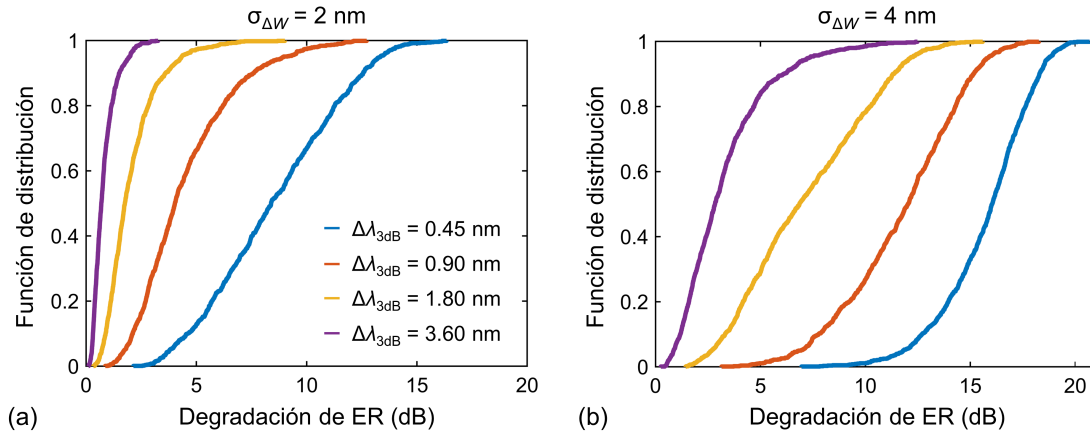
Figura 4.11. Análisis del impacto del ruido de fase en filtros sinusoidales con diferentes anchos de banda: funciones de distribución acumuladas correspondientes a la degradación de ER para desviaciones típicas (a) \sigma_{\Delta W} = 2 nm y (b) \sigma_{\Delta W} = 4 nm. Cada color identifica un ancho de banda nominal distinto, siendo todos los filtros diseñados para la configuración con núcleo Si-wire y polarización TM. Se han simulado un total de 1000 realizaciones aleatorias por caso, con una longitud de correlación L_{c,\Delta W} = 15 \mu\text{m} .
