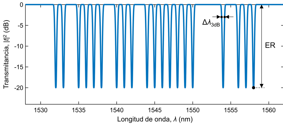
Figura 3.17. Transmitancia espectral objetivo del filtro astrofónico a diseñar, formado por 20 notches en posiciones arbitrarias.
