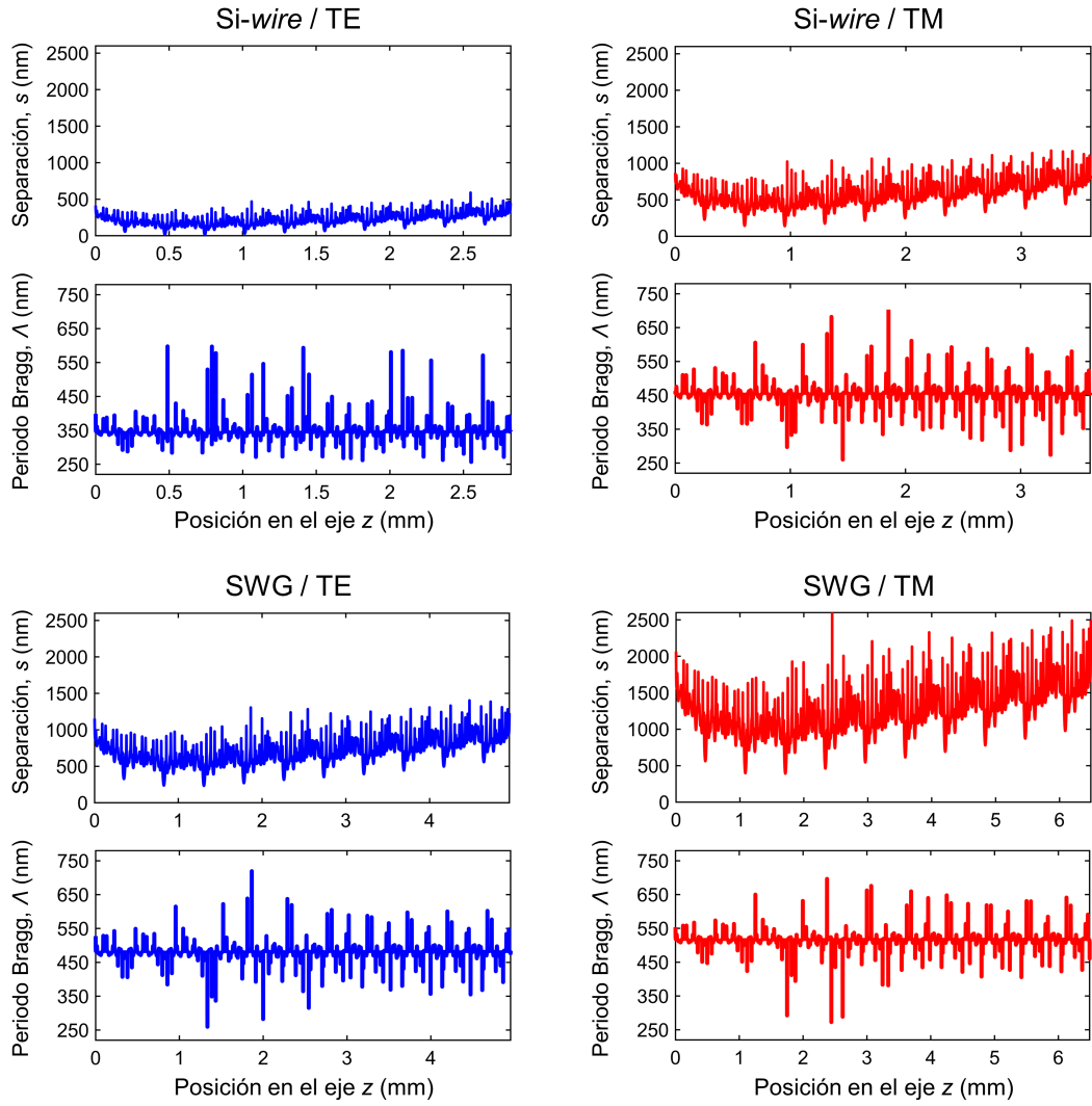
Figura 3.19. Perfiles de separación lateral y periodo Bragg de filtros astrofotónicos para las diferentes configuraciones de filtro. Los resultados se corresponden con la especificación espectral de filtro mostrada en la tabla 3.6.
