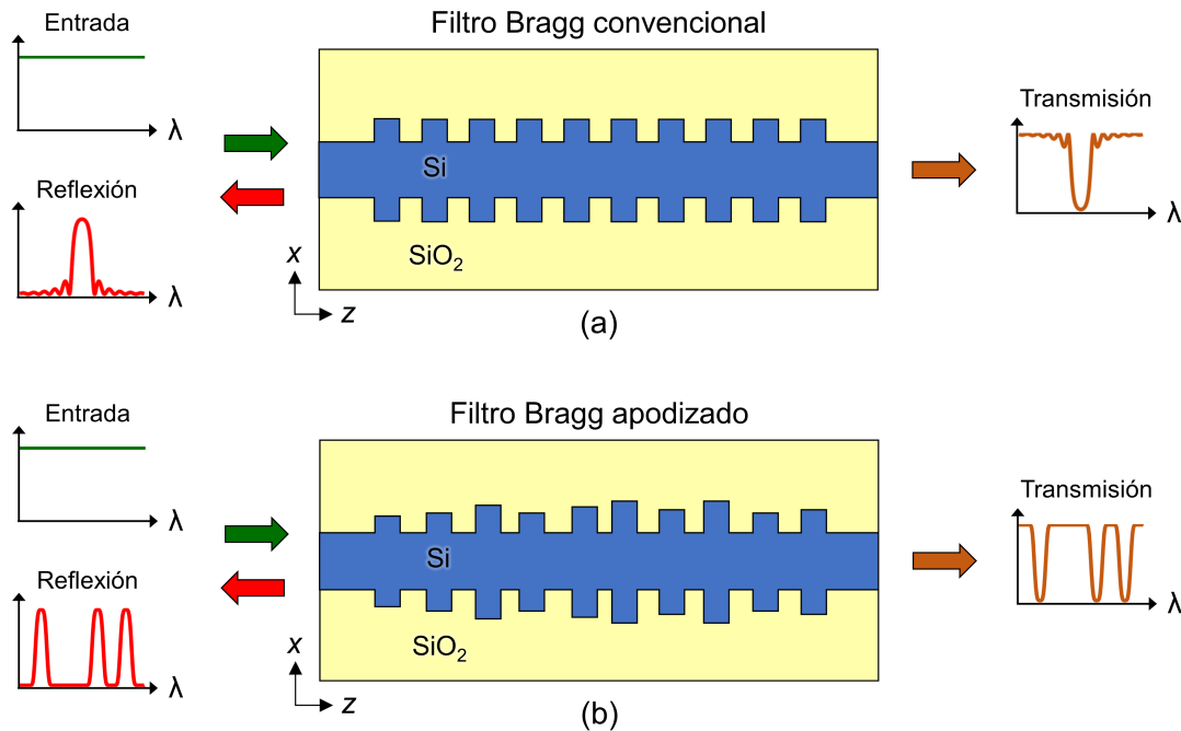
Figura 1.3. Representación esquemática 2D (vista superior) de (a) filtro Bragg convencional y (b) filtro Bragg apodizado en la plataforma SOI. Los filtros Bragg convencionales (o no apodizados) son estructuras completamente periódicas y sintetizan un único pico de reflexión en su respuesta espectral. Los filtros Bragg apodizados presentan un perfil de índice de refracción aperiódico y permiten implementar respuestas con formas espectrales arbitrarias.
