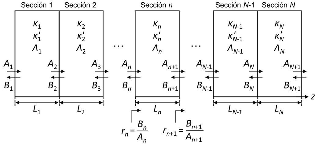
Figura 2.15. Representación del modelo de filtro Bragg apodizado en que se basa el TMM. El filtro Bragg apodizado se divide en N secciones de filtro Bragg no apodizado, cada una con coeficiente de acoplo \kappa_n , coeficiente de autoacoplo \kappa'_n , periodo \Lambda_n y longitud L_n . Las amplitudes de los modos forward y backward a la entrada de cada sección n se denotan como A_n y B_n , respectivamente, con r_n = B_n/A_n siendo el coeficiente de reflexión total visto desde dicho interfaz.
