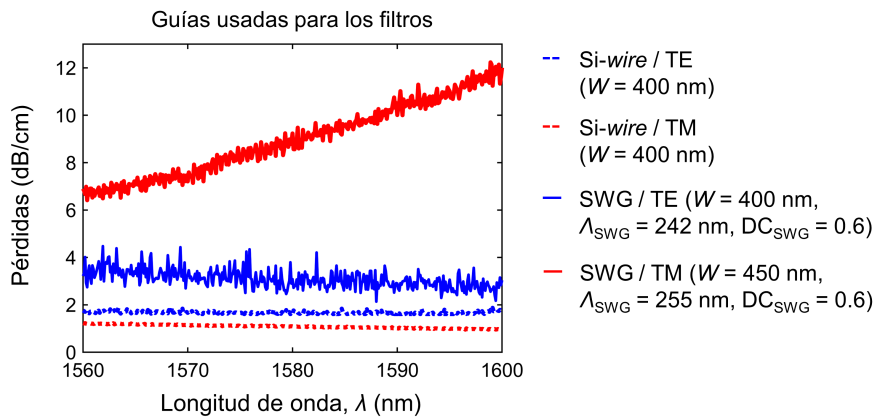
Figura 3.28. Estimación de las pérdidas de propagación de las guías utilizadas como núcleo en las distintas configuraciones de filtro. Junto a la figura se recuerdan las dimensiones de cada una de las guías.
