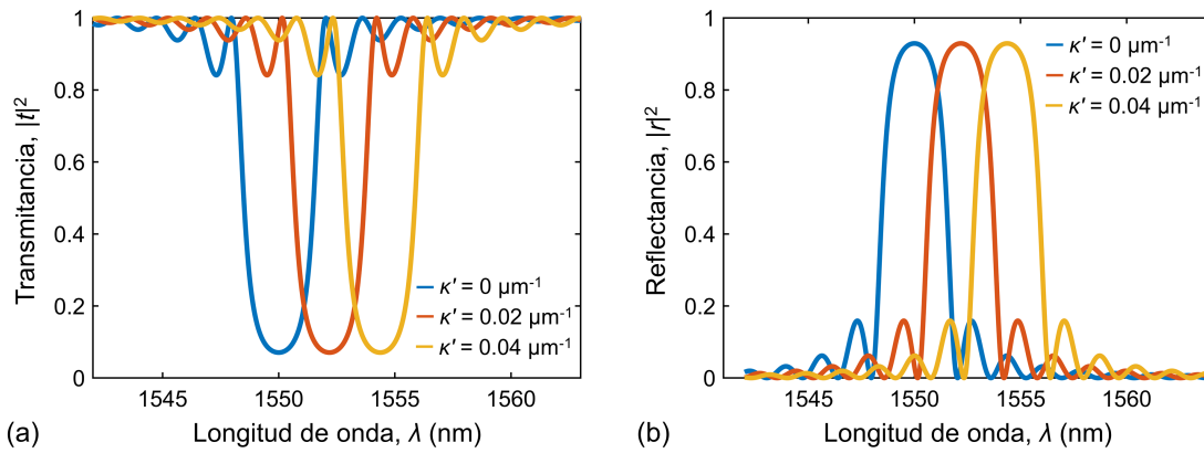
Figura 2.10. (a) Transmitancia y (b) reflectancia de un filtro Bragg no apodizado para diferentes coeficientes de autoacoplo: \kappa' = 0 \mu\text{m}^{-1} (azul), \kappa' = 0.02 \mu\text{m}^{-1} (rojo), y \kappa' = 0.04 \mu\text{m}^{-1} (amarillo). Parámetros fijos en todas las curvas: \lambda_0 = 1550 \text{ nm} , n_{g,u}(\lambda_0) = 3.5 , \kappa = 0.01 \mu\text{m}^{-1} , y L = 200 \mu\text{m} .
