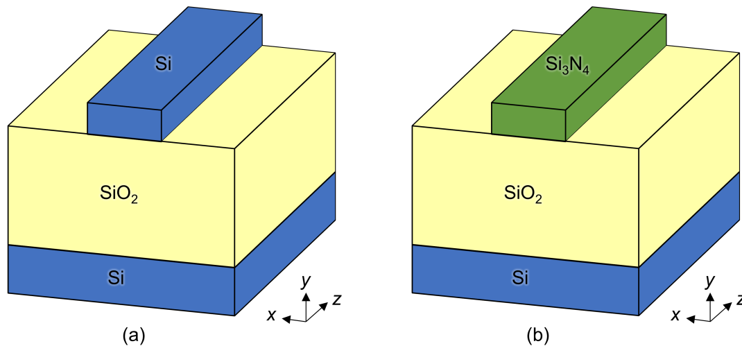
Figura 1.2. Representación esquemática 3D de guías de onda típicas (a) en la plataforma SOI y (b) en la plataforma de nitruro de silicio. Opcionalmente, en algunas ocasiones se deposita un recubrimiento de dióxido de silicio en la parte superior de las guías, también denominado cladding .
