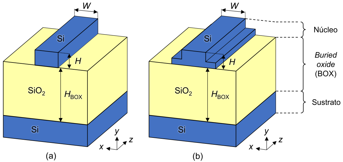
Figura 3.1. Representación esquemática 3D de (a) guía Si-wire y (b) guía rib en la plataforma SOI, junto con la denominación de las diferentes capas de materiales a la derecha. De forma adicional, algunas veces se incluye un recubrimiento de dióxido de silicio en la parte superior de la estructura (encima del núcleo), también llamado cladding . A la longitud de onda \lambda = 1.55 \mu\text{m} los índices de refracción de silicio y dióxido de silicio son, respectivamente, n_{\text{Si}} \approx 3.48 y n_{\text{SiO}_2} \approx 1.44 .
