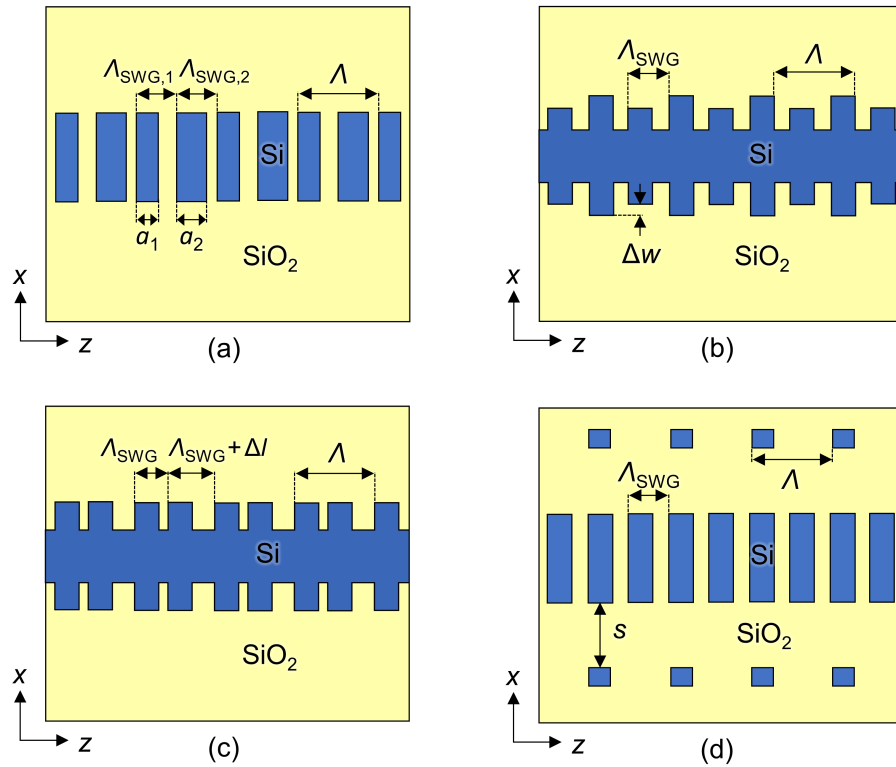
Figura 3.4. Representación esquemática 2D (vista superior) de filtros Bragg en tecnología SOI basados en estructuras SWG: (a) filtros con núcleo segmentado, usando dos periodos de tamaño SWG y diferentes dimensiones por cada periodo Bragg; (b) filtros basados en guías con corrugaciones de tamaño SWG, modulando la diferencia de anchura entre corrugaciones SWG consecutivas; (c) filtros basados en guías con corrugaciones de tamaño SWG, usando diferentes longitudes para cada corrugación SWG; (d) filtros con núcleo segmentado SWG y perturbación del campo evanescente, insertando segmentos de silicio de forma paralela a la guía SWG central.
