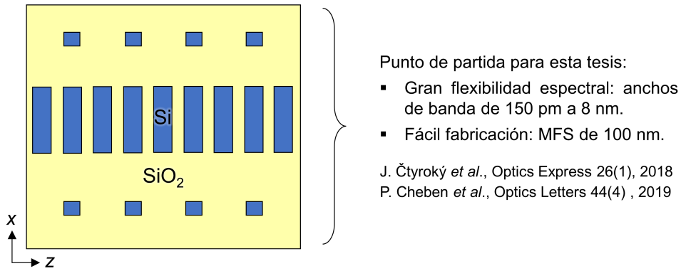
Figura 1.4. Representación esquemática 2D (vista superior) de la topología de filtro Bragg no apodizado propuesta en [47] y evaluada experimentalmente en [48], que sirve como punto de partida para esta tesis.
