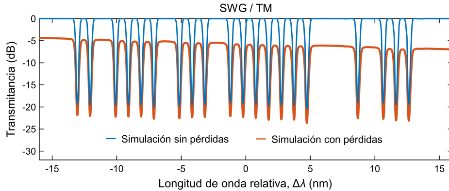
Figura 3.35. Transmisión simulada del filtro astrofotónico para núcleo SWG y polarización TM, calculada mediante el TMM, sin pérdidas de propagación (azul) y con las pérdidas de propagación estimadas en los resultados experimentales (rojo). El eje de abscisas se ha definido como la longitud de onda relativa con respecto del notch número 11 de izquierda a derecha.
