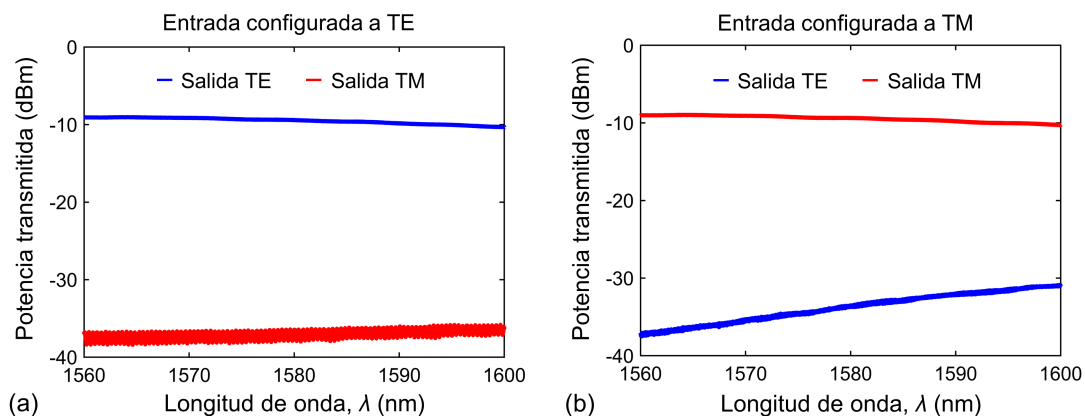
Figura 3.25. Potencia recibida en el fotodiodo de salida al conectar directamente la fibra óptica de entrada y el objetivo de microscopio, configurando los controladores de polarización de la entrada para: (a) excitación con polarización TE y (b) excitación con polarización TM. En azul y rojo se muestra la potencia recibida en el fotodiodo al ajustar el prisma polarizador de salida para permitir pasar únicamente luz TE o luz TM, respectivamente. La potencia de entrada del láser es -1 dBm.
