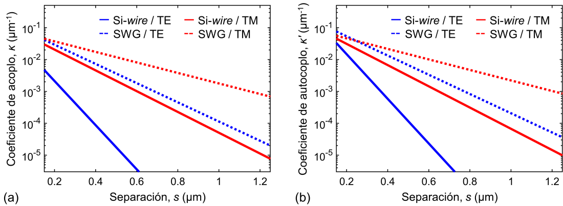
Figura 3.10. Coeficientes de (a) acoplo y (b) autoacoplo del filtro en función de la separación de los segmentos laterales. Nótese que el eje vertical se representa en escala logarítmica.
