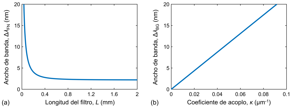
Figura 2.11. Variación del ancho de banda de un filtro Bragg no apodizado en función de (a) su longitud y (b) su coeficiente de acoplo. Parámetros fijos en ambas curvas: \lambda_0 = 1550 nm, y n_{\text{g,u}}(\lambda_0) = 3.5 . En la curva (a) se representa el ancho de banda entre primeros nulos de reflexión con \kappa = 0.01 \mu\text{m}^{-1} , mientras que en la curva (b) se representa el ancho de banda del bandgap ( L \rightarrow \infty ).
