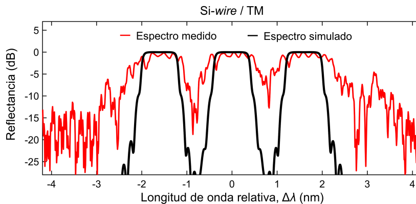
Figura 3.37. Reflectancia medida para el filtro flat-top de tres bandas con núcleo Si-wire y polarización TM (rojo), junto con la reflectancia simulada mediante el TMM (negro). Para comparar ambas respuestas, el eje vertical del espectro medido ha sido normalizado a un máximo de 0 dB. El eje de abscisas se ha definido como la longitud de onda relativa con respecto de la banda central del filtro.
