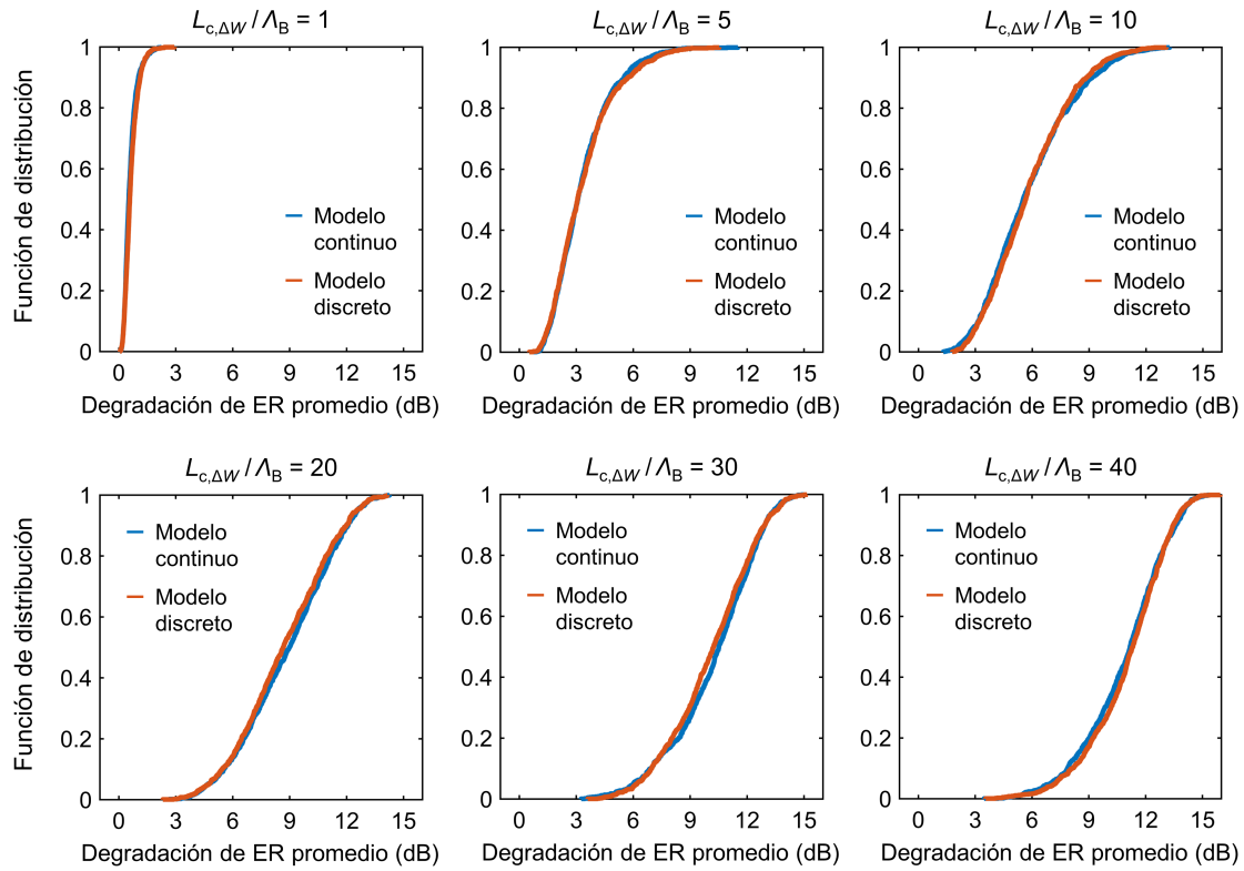
Figura 4.9. Validación del modelo de ruido de fase discreto mediante simulación de un filtro con tres notches: funciones de distribución acumuladas correspondientes a la degradación del ER promedio de los tres notches del filtro para diferentes longitudes de correlación L_{c,\Delta W} , obtenidas con el modelo continuo (azul) y con el modelo discreto (rojo). Se han simulado un total de 1000 realizaciones aleatorias por caso. La desviación típica del error de anchura se ha elegido como \sigma_{\Delta W} = 4 nm.
