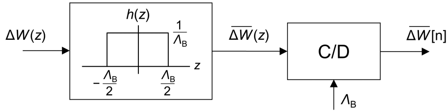
Figura 4.3. Procesado de señal aplicado sobre el error de anchura continuo, \Delta W(z) , para calcular el error de anchura promedio en cada periodo Bragg, \overline{\Delta W}[n] .
