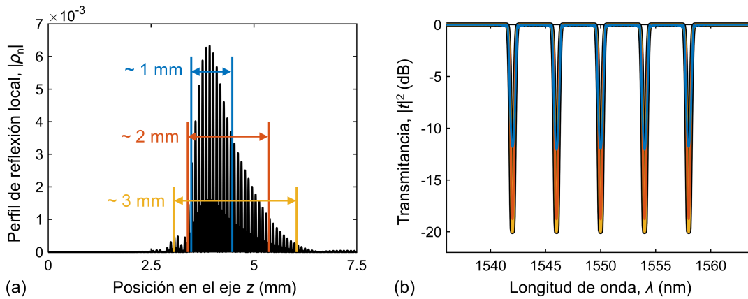
Figura 2.20. Representación del impacto de aplicar diferentes ventanas de truncamiento sobre el perfil de reflexión local. Como ejemplo, se ha utilizado un filtro objetivo con un espectro de transmisión formado por cinco notches a longitudes de onda arbitrarias, con: \lambda_0 = 1550 nm, \Lambda_B = 500 nm, y n_{g,u}(\lambda_0) = 3.5 . (a) Módulo del perfil de reflexión local \rho_n con respecto a la posición espacial z = n\Lambda_B , calculado mediante el algoritmo LP para N = 15\,000 periodos. También se muestran las ventanas de truncamiento usadas para obtener el perfil de reflexión acortado \tilde{\rho}_n , con longitudes de filtro de aproximadamente 1 mm (azul), 2 mm (rojo) y 3 mm (amarillo). (b) Transmitancia objetivo (negro) y transmitancia calculada mediante el algoritmo LA para los diferentes perfiles de reflexión acortados: 1 mm (azul), 2 mm (rojo) y 3 mm (amarillo).
