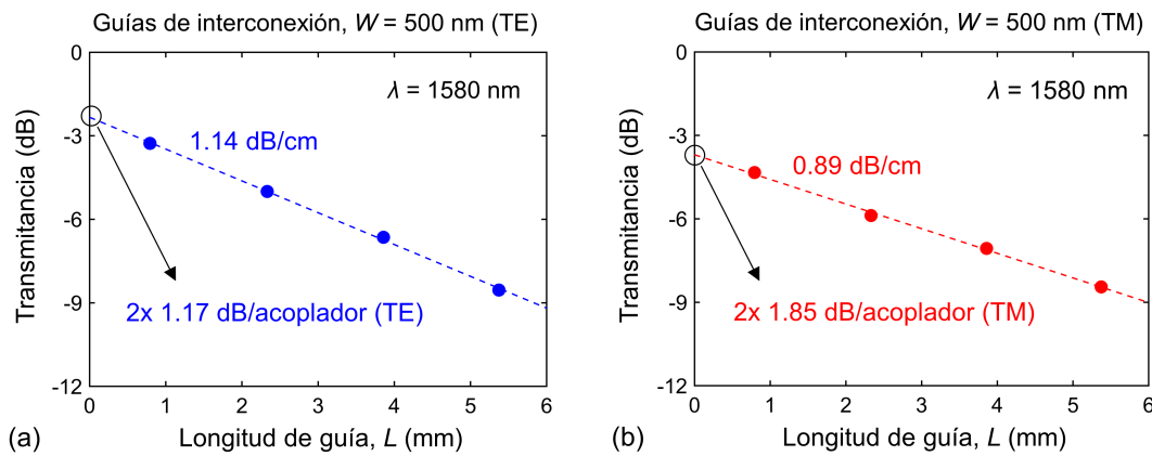
Figura 3.26. Transmitancia medida para las estructuras de prueba basadas en guías interconexión de anchura 500 nm a la longitud de onda \lambda = 1580 nm, con (a) polarización TE y (b) polarización TM. La interpolación lineal representada en línea discontinua ilustra la aplicación del método de cutback , que permite estimar tanto las pérdidas de propagación de las guías como las pérdidas de los edge couplers .
