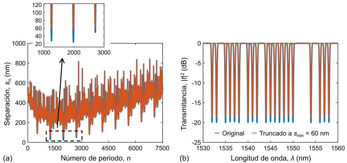
Figura 4.17. Filtro astrofotónico basado en guía Si-wire de anchura W = 600 nm y polarización TM: (a) perfil de separación de los segmentos laterales; (b) transmitancia espectral sintetizada, obtenida mediante el TMM. Las curvas de color azul representan el diseño nominal, mientras que las de color rojo se corresponden con el caso de truncar las separaciones de los segmentos laterales a un mínimo de 60 nm, por las restricciones del proceso de fabricación en la práctica. En la parte superior izquierda se muestra la vista ampliada del perfil de separación en la zona donde se realiza el truncamiento.
