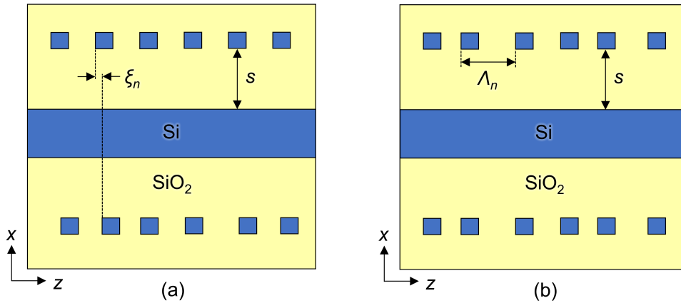
Figura 5.1. Representación esquemática 2D (vista superior) de filtros Bragg con perturbación del campo evanescente y núcleo Si-wire basados en esquemas de apodización alternativos: (a) modulación del desalineamiento entre los segmentos a cada lado de la guía, \xi_n ; (b) modulación de la fase del grating , es decir, de la longitud del periodo Bragg \Lambda_n . En ambos casos, la separación s de los segmentos laterales se mantiene constante a lo largo del filtro.
