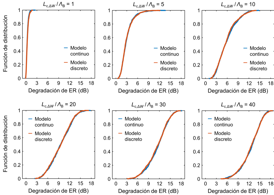
Figura 4.7. Validación del modelo de ruido de fase discreto mediante simulación de un filtro con apodización sinusoidal: funciones de distribución acumuladas correspondientes a la degradación de ER del filtro para diferentes longitudes de correlación L_{c,\Delta W} , obtenidas con el modelo continuo (azul) y con el modelo discreto (rojo). Se han simulado un total de 1000 realizaciones aleatorias por caso. La desviación típica del error de anchura se ha elegido como \sigma_{\Delta W} = 4 nm.
