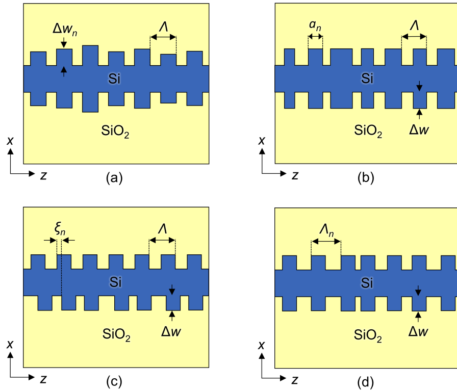
Figura 3.5. Representación esquemática 2D (vista superior) de filtros Bragg apodizados en tecnología SOI mediante diferentes técnicas de apodización: (a) modulación de la anchura de corrugación \Delta w_n ; (b) modulación del ciclo de trabajo DC_n = a_n / \Lambda ; (c) modulación del desalineamiento entre las corrugaciones de cada lado \xi_n ; y (d) modulación de la fase del grating , es decir, de la longitud del periodo Bragg \Lambda_n .
