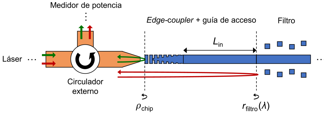
Figura 3.38. Representación esquemática del modelo utilizado para estudiar los problemas observados en los resultados experimentales de los filtros flat-top . Los tramos de fibras ópticas se muestran en naranja, mientras que los tramos de guías de silicio dentro del chip se muestran en azul. Las flechas verdes y rojas representan las dos contribuciones principales de la señal reflejada recibida en el medidor de potencia.
