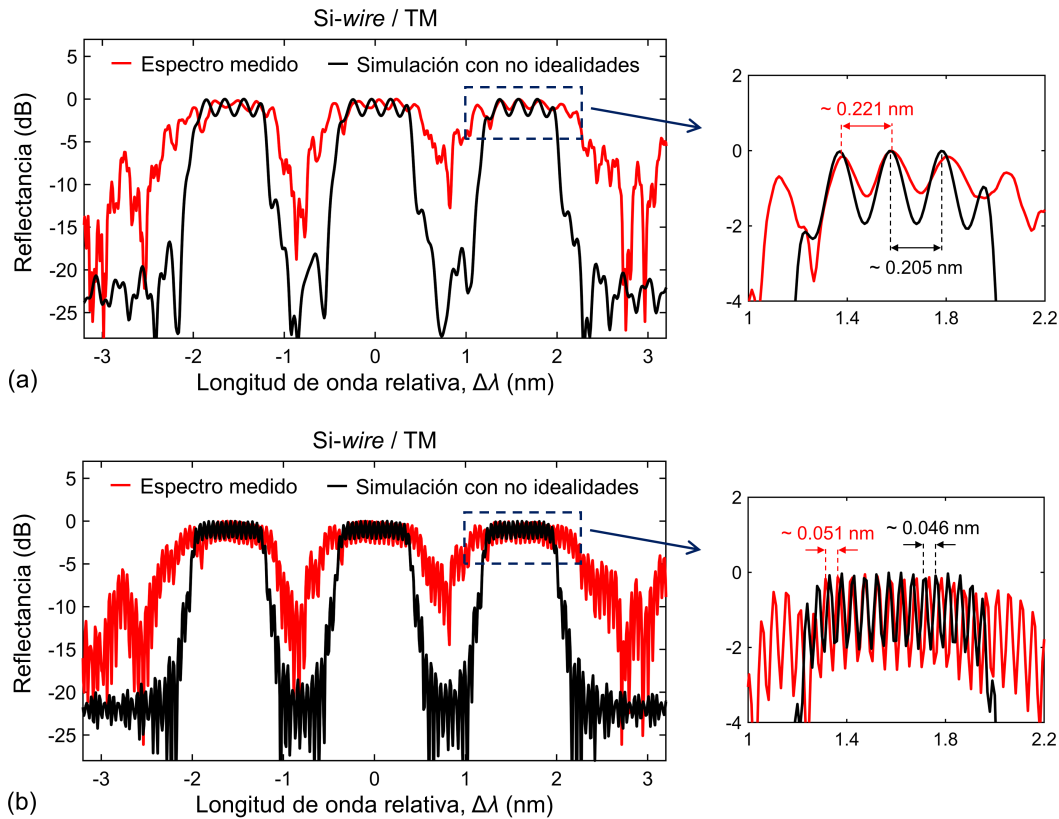
Figura 3.39. Reflectancia medida para el filtro flat-top de tres bandas con núcleo Si-wire y polarización TM (rojo), excitando el filtro desde el edge-coupler (a) de un extremo y (b) del extremo opuesto. Junto a las curvas experimentales, se representan las simulaciones del filtro basadas en el esquema propuesto en la figura 3.38 (negro). Para comparar ambas respuestas, el eje vertical de los dos espectros ha sido normalizado a un máximo de 0 dB. El eje de abcisas se ha definido como la longitud de onda relativa con respecto de la banda central del filtro. A la derecha se muestra la vista ampliada de una de las bandas.
