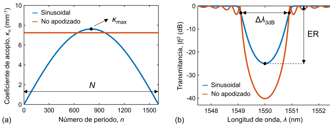
Figura 3.11. Comparativa entre filtro con apodización sinusoidal (azul) y filtro no apodizado (rojo): (a) perfil de coeficiente de acoplo y (b) transmitancia espectral sintetizada, calculada mediante el TMM. Ambos filtros presentan la misma longitud y el mismo ancho de banda a 3 dB, y se basan en la configuración con núcleo Si-wire y polarización TM. Parámetros de diseño del filtro sinusoidal: \kappa_{\max} = 7.62 \text{mm}^{-1} y N = 1608 periodos. Parámetros de diseño del filtro no apodizado: \kappa = 7.24 \text{mm}^{-1} y N = 1608 periodos.
