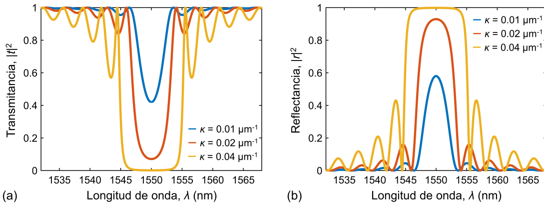
Figura 2.8. (a) Transmitancia y (b) reflectancia de un filtro Bragg no apodizado para diferentes coeficientes de acoplo: \kappa = 0.01 \mu\text{m}^{-1} (azul), \kappa = 0.02 \mu\text{m}^{-1} (rojo), y \kappa = 0.04 \mu\text{m}^{-1} (amarillo). Parámetros fijos en todas las curvas: \lambda_0 = 1550 nm, n_{g,u}(\lambda_0) = 3.5 , y L = 100 \mu\text{m} .
