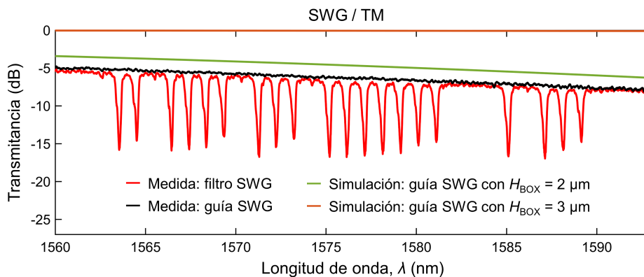
Figura 3.34. Comparación de transmitancia medida para el filtro astrofotónico con núcleo SWG y polarización TM (rojo), transmitancia medida para una guía SWG de igual longitud (negro), y transmitancia simulada para una guía SWG de igual longitud y espesores de BOX de 2 \mu\text{m} (verde) y 3 \mu\text{m} (naranja). En las simulaciones se han considerado los errores de fabricación previamente estimados en las dimensiones de la guía. En las curvas experimentales se han descontado previamente las pérdidas del sistema de medida, de los edge-couplers y de las guías de interconexión.
