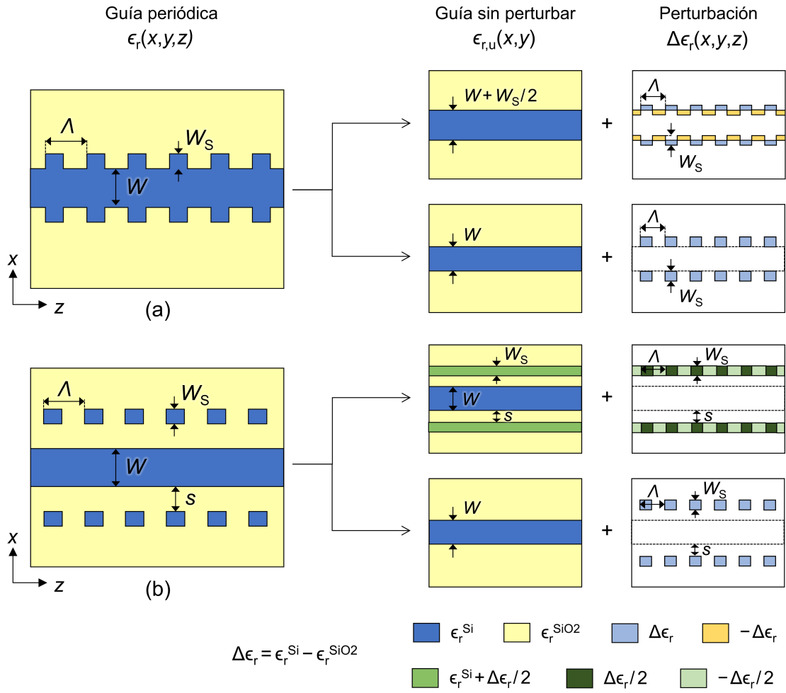
Figura 2.6. Representación esquemática 2D (vista superior) de una estructura periódica como la superposición de una guía uniforme y una perturbación periódica para diferentes geometrías de filtro Bragg no apodizado en la plataforma SOI: (a) guía con corrugaciones laterales y (b) guía con perturbación del campo evanescente. Para cada caso, se ilustran dos posibles definiciones de guía sin perturbar y perturbación periódica.
