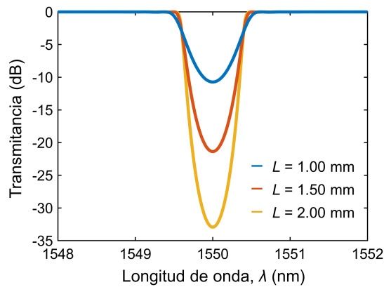
Figura 4.13. Análisis del impacto del ruido de fase en filtros sinusoidales con diferentes ER: comparación de las respuestas espectrales nominales, obtenidas mediante el TMM. Cada color identifica un diseño de filtro distinto, siendo todos los filtros diseñados para la configuración con núcleo Si-wire y polarización TM.
