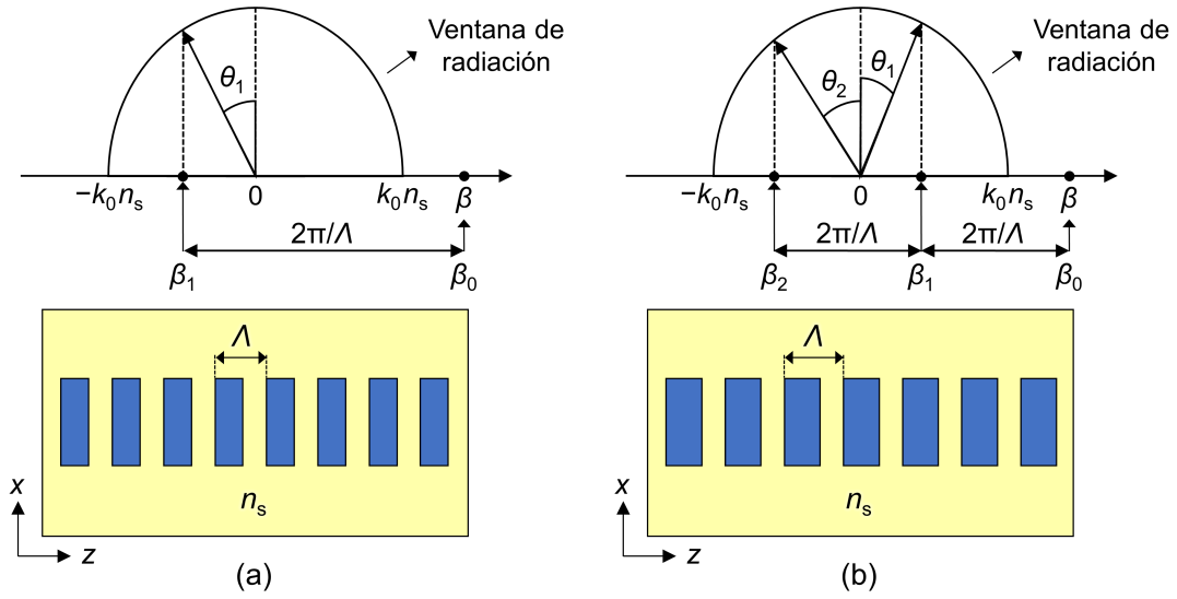
Figura 2.2. Representación gráfica de la condición de radiación en una estructura periódica, para dos situaciones distintas: (a) radiación de únicamente un armónico ( m = 1 ); (b) radiación de dos armónicos simultáneamente ( m = 1 y m = 2 ). En este ejemplo, se ilustra el fenómeno de radiación en el medio lateral, pero también puede darse en los medios superior e inferior.
