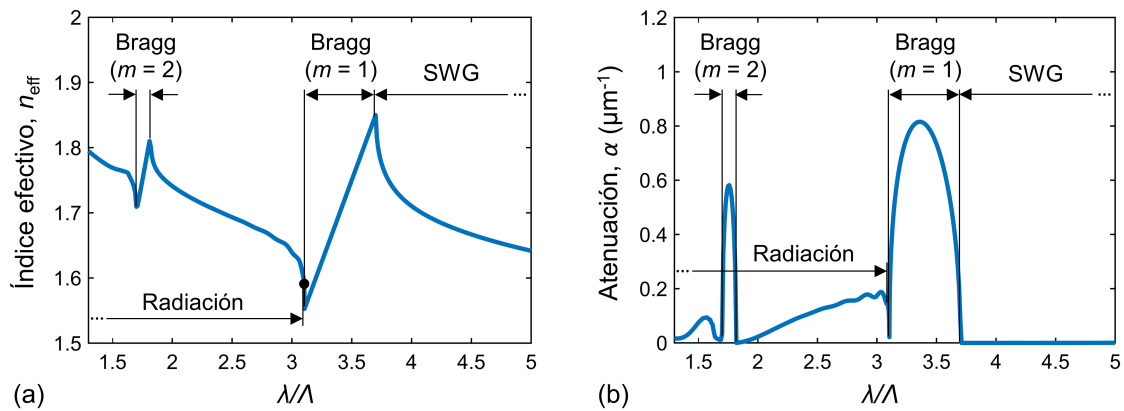
Figura 2.4. Variación de (a) índice efectivo y (b) constante de atenuación del modo Floquet-Bloch en función del cociente entre la longitud de onda y el periodo de la estructura. Junto a las gráficas se identifican las diferentes zonas de trabajo de la guía periódica. Los datos corresponden a la misma estructura que se ha analizado en la figura 2.3.
