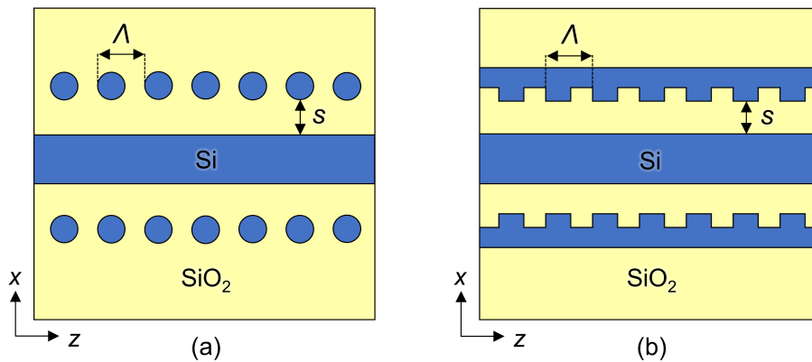
Figura 3.3. Representación esquemática 2D (vista superior) de filtros Bragg en tecnología SOI basados perturbación del campo evanescente: (a) insertando segmentos laterales de silicio junto a una guía Si-wave, y (b) usando guías con corrugaciones laterales paralelas a la guía Si-wave central.
