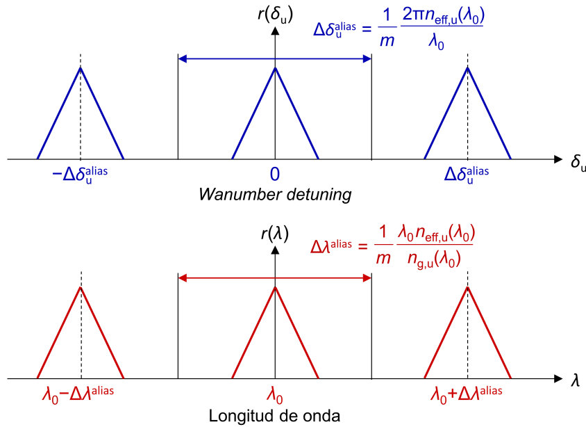
Figura A.1. Representación esquemática de la periodicidad de la respuesta espectral sintetizada mediante los algoritmos LP y LA, en términos de (a) wavenumber detuning y (b) longitud de onda.
