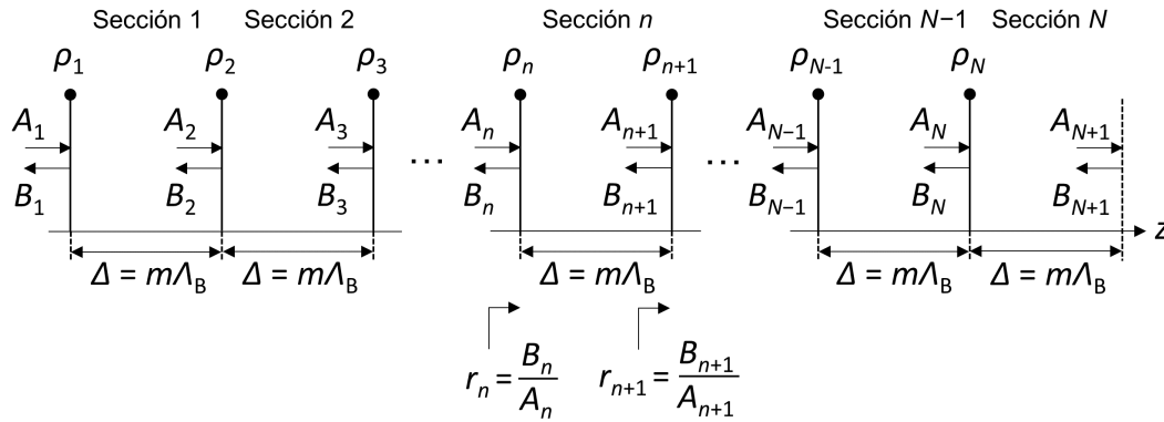
Figura 2.17. Representación del modelo de filtro Bragg apodizado en que se basan los algoritmos LP y LA. El filtro Bragg apodizado se divide en N secciones de filtro uniforme, donde cada sección se forma como la combinación de un reflector local discreto con coeficiente de reflexión \rho_n , con n siendo el número de sección, y una línea de transmisión de longitud \Delta . La longitud de sección \Delta se corresponde con una agrupación de m periodos Bragg, con longitud de periodo \lambda_B (para los filtros de esta tesis, m = 1 ). Las amplitudes de los modos forward y backward a la entrada de cada sección n se denotan como A_n y B_n , respectivamente, con r_n = B_n/A_n siendo el coeficiente de reflexión total visto desde dicho interfaz
