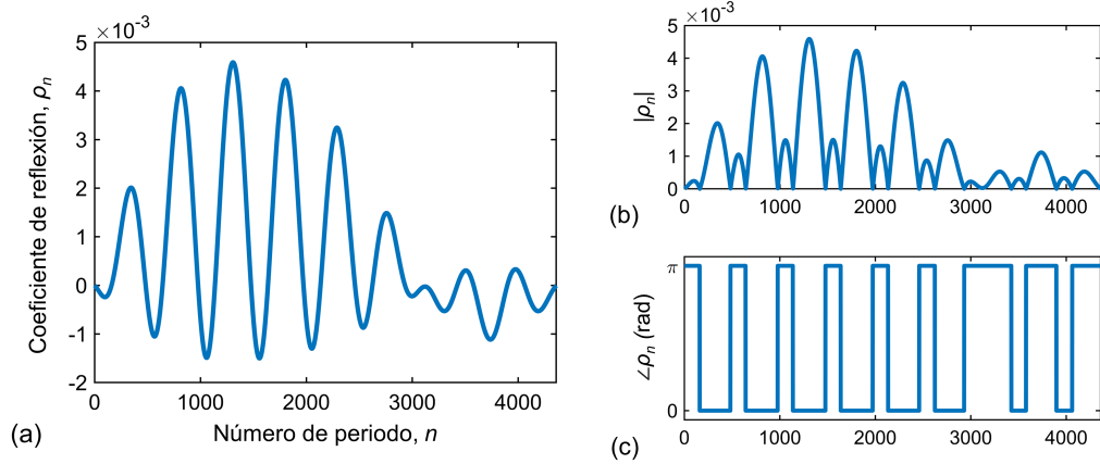
Figura 3.15. (a) Perfil de coeficiente de reflexión local para uno de los filtros flat-top multicanal diseñados, incluyendo (b) módulo y (c) fase. El resultado corresponde a un filtro flat-top de tres canales para la configuración con núcleo Si-wire y polarización TM, con los siguientes parámetros objetivo: r_{\max} = 0.995 , \Delta\lambda_{3\text{dB}} = 0.8 \text{ nm} y \Delta\lambda_{\text{canal}} = 1.6 \text{ nm} . El perfil \rho_n mostrado es el resultante de haber aplicado el algoritmo LP sobre la respuesta objetivo y utilizar una ventana de truncamiento para reducir la longitud del filtro.
