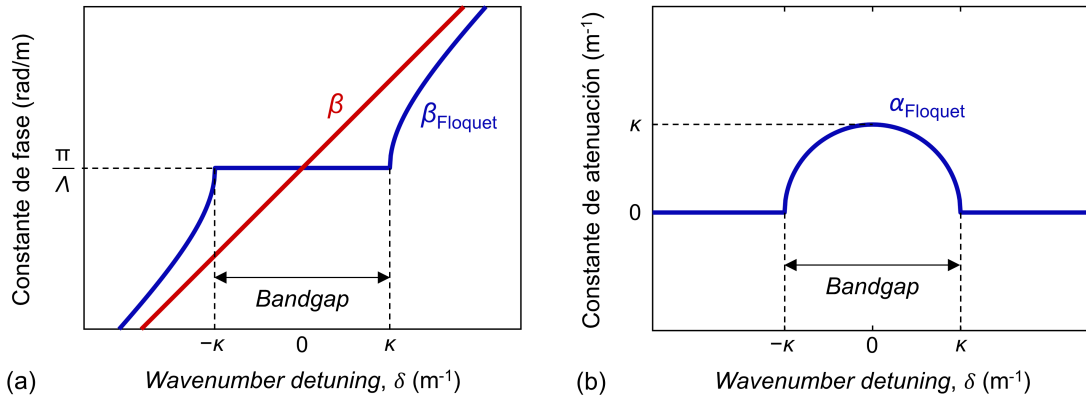
Figura 2.7. Representación esquemática de la evolución con respecto al wavenumber detuning de: (a) constante de fase del modo Floquet-Bloch de la guía periódica (azul) y constante de fase de la guía perturbada (rojo); (b) constante de atenuación del modo Floquet-Bloch de la guía periódica.
