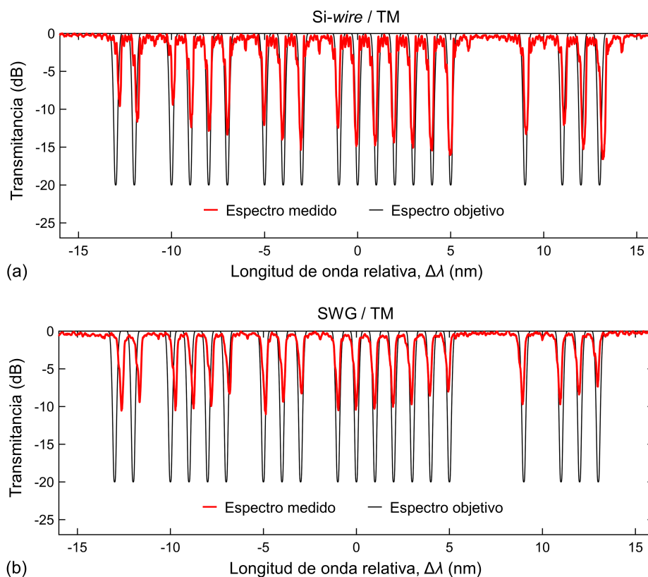
Figura 3.32. Respuesta en transmitancia medida para los filtros astrofotónicos, normalizadas por las pérdidas de inserción del núcleo (sin segmentos laterales), con las configuraciones de filtro: (a) Si-wire /TM, y (b) SWG/TM. El eje de abcisas se ha definido como la longitud de onda relativa con respecto del notch número 11 de izquierda a derecha.
