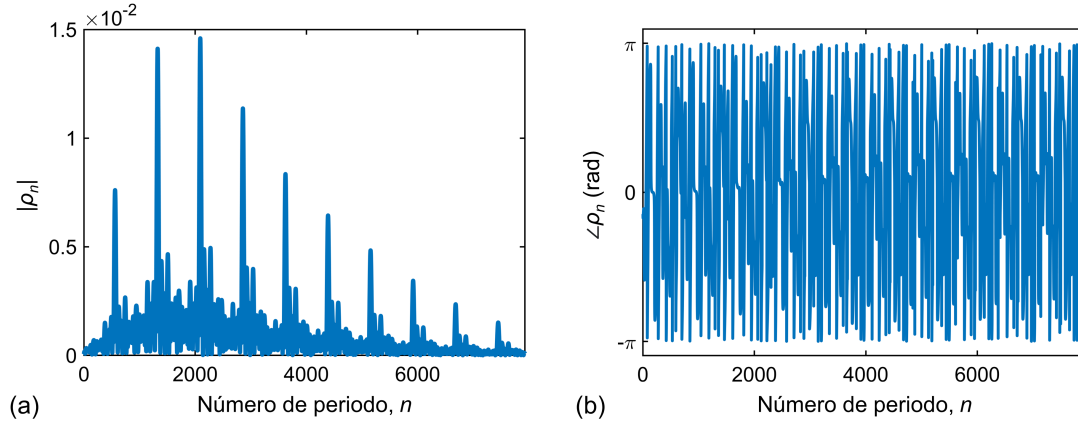
Figura 3.18. Perfil de coeficiente de reflexión local para uno de los filtros astrofotónicos diseñados: (a) módulo y (b) fase. El resultado corresponde a la configuración con núcleo Si-wire y polarización TM, con la especificación de filtro resumida en la tabla 3.6. El perfil \rho_n mostrado es el resultante de haber aplicado el algoritmo LP sobre la respuesta objetivo y utilizar una ventana de truncamiento para reducir la longitud del filtro.
