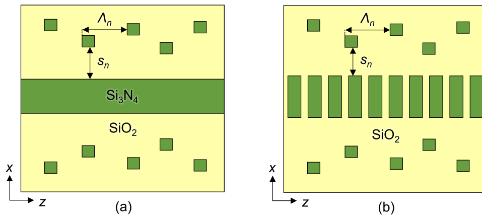
Figura 5.2. Representación esquemática 2D (vista superior) de las estructuras Bragg apodizadas estudiadas en esta tesis adaptadas al caso de la plataforma de nitruro de silicio, con (a) núcleo Si-wire y (b) núcleo SWG.
