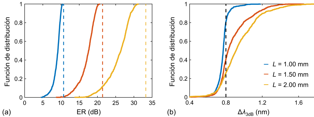
Figura 4.14. Análisis del impacto del ruido de fase en filtros sinusoidales con diferentes ER: funciones de distribución acumuladas de (a) ER y (b) ancho de banda a 3 dB. Cada color identifica un diseño de filtro distinto, siendo todos los filtros diseñados para la configuración con núcleo Si-wire y polarización TM. Las líneas verticales discontinuas indican los correspondientes valores nominales, teniéndose el mismo valor nominal de ancho de banda a 3 dB en los tres filtros. Se han simulado un total de 1000 realizaciones aleatorias por caso, con una desviación típica \sigma_{\Delta W} = 2 nm y una longitud de correlación L_{c,\Delta W} = 15 \mu m.
