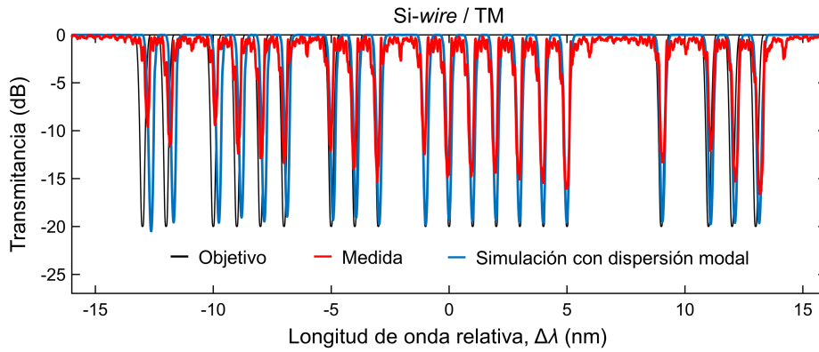
Figura 3.36. Comparación de transmitancia objetivo del filtro astrofotónico (negro), transmitancia medida para el filtro astrofotónico con núcleo Si-wire y polarización TM (rojo), y transmitancia simulada para el filtro astrofotónico con núcleo Si-wire y polarización TM considerando el efecto de la dispersión modal (azul). El eje de abscisas se ha definido como la longitud de onda relativa con respecto del notch número 11 de izquierda a derecha.
