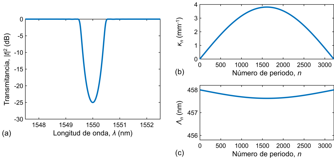
Figura 4.6. Diseño nominal del filtro con apodización sinusoidal utilizado para comparar los modelos de ruido de fase discreto y continuo: (a) transmitancia espectral sintetizada, obtenida mediante el TMM; (b) perfil de coeficiente de acoplo; (c) perfil de periodo Bragg.
