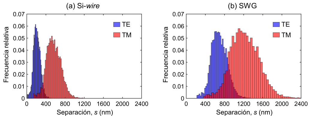
Figura 3.20. Distribuciones de frecuencia relativa de las separaciones de los segmentos laterales para los filtros astrofotónicos diseñados: (a) comparativa para filtros con núcleo Si-wire y (b) comparativa para filtros con núcleo SWG. Todos los histogramas se han calculado utilizando el mismo número de intervalos.
