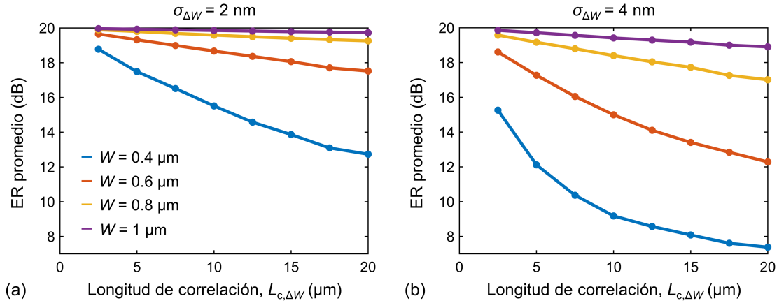
Figura 4.16. Análisis del impacto del ruido de fase en filtros no apodizados con diferentes anchuras de guía: ER promedio en función de la longitud de correlación L_{c,\Delta W} para desviaciones típicas (a) \sigma_{\Delta W} = 2 \text{ nm} y (b) \sigma_{\Delta W} = 4 \text{ nm} . Los puntos muestran los valores de longitud de correlación simulados. Cada color identifica el diseño correspondiente a una anchura de guía, siendo todos los filtros diseñados para la configuración con núcleo Si-wire y polarización TM. Se han simulado un total de 1000 realizaciones aleatorias por caso.
