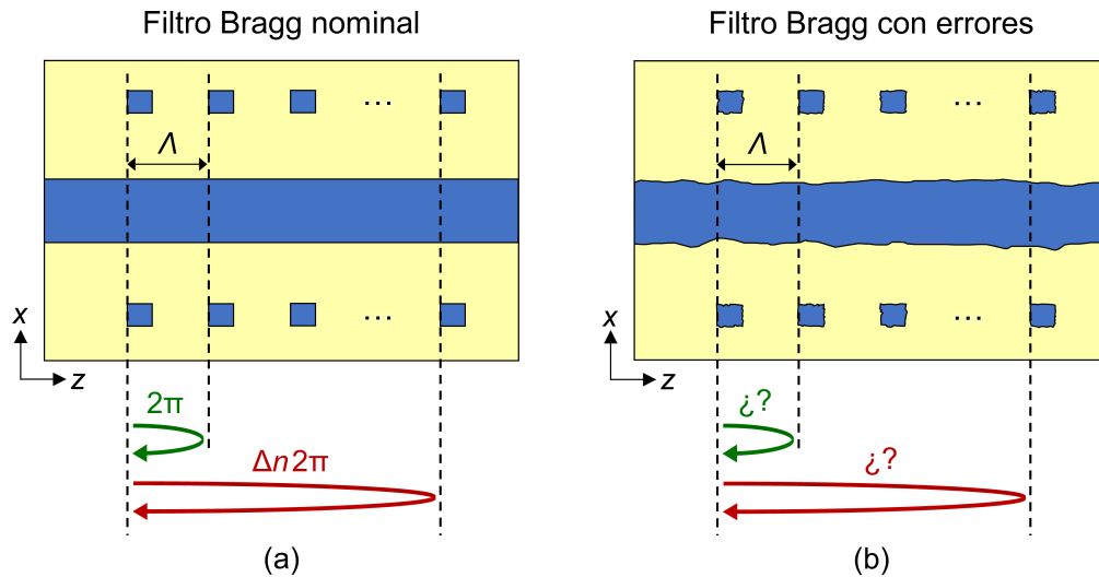
Figura 4.1. Representación esquemática 2D (vista superior) de un filtro Bragg no apodizado, (a) con dimensiones nominales y (b) con variaciones aleatorias causadas por las imperfecciones de la fabricación. Mientras en el caso ideal las reflexiones parciales en diferentes periodos del filtro interfieren entre sí de forma constructiva, los errores de fabricación en las estructuras reales hacen que estas diferencias de fase entre reflexiones parciales presenten un carácter aleatorio, pudiendo distorsionar la respuesta del filtro.
