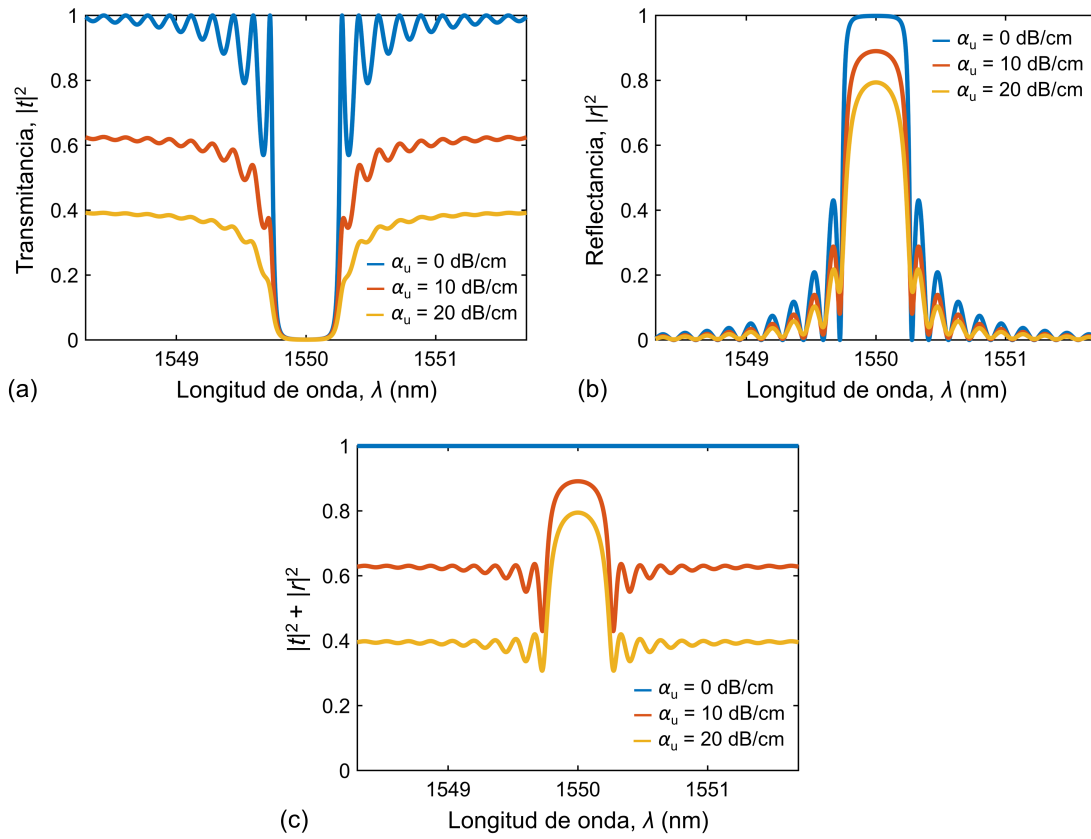
Figura 2.14. (a) Transmitancia, (b) reflectancia y (c) suma de transmitancia y reflectancia para un filtro Bragg no apodizado con diferentes pérdidas de propagación: \alpha_u = 0 dB cm -1 (azul), \alpha_u = 10 dB cm -1 (rojo), y \alpha_u = 20 dB cm -1 (amarillo). Parámetros fijos en todas las curvas: \lambda_0 = 1550 nm, n_{g,u}(\lambda_0) = 3.5 , \kappa = 0.002 \mu\text{m}^{-1} , y L = 2 mm.
