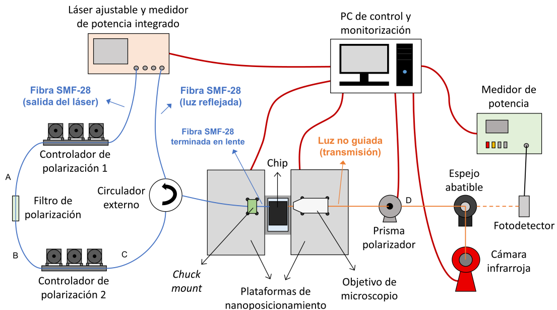
Figura 3.23. Representación esquemática del montaje de medida usado para caracterizar las estructuras fabricadas. Las líneas azules representan fibras ópticas, las líneas naranjas son tramos en los que la luz se propaga de forma no guiada, y las líneas rojas muestran conexiones eléctricas con el PC del laboratorio. Todas las fibras ópticas del montaje son SMF-28, es decir, no mantenedoras de la polarización.
