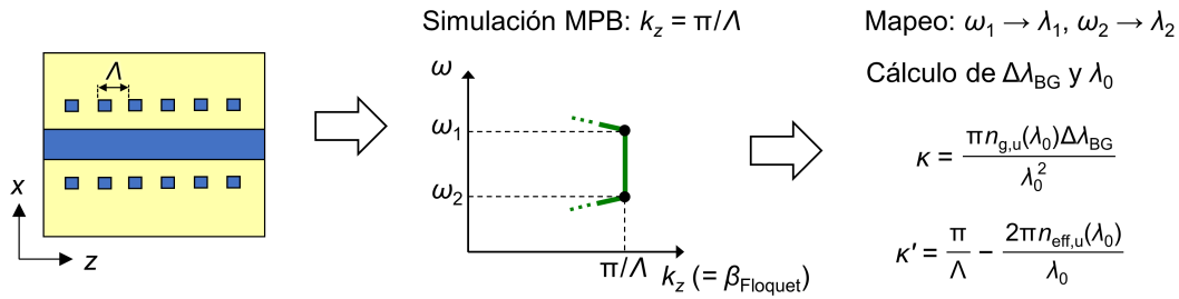
Figura 2.13. Representación esquemática del procedimiento de cálculo de los coeficientes de acoplo de un grating usando la herramienta de simulación MPB.
