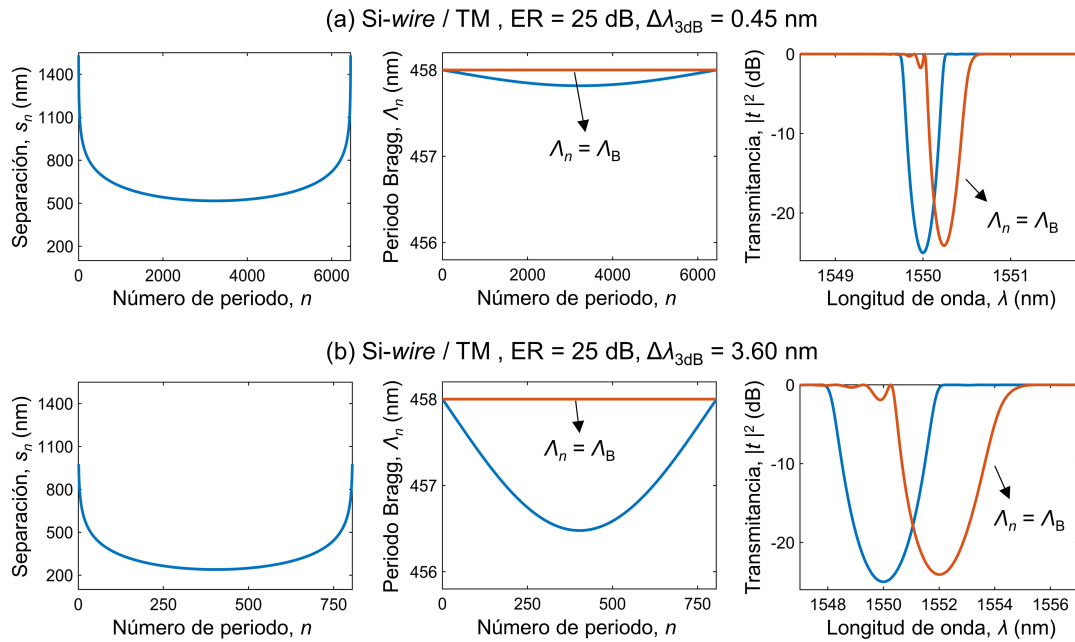
Figura 3.12. Perfil de separación lateral, perfil de periodo Bragg y transmitancia espectral sintetizada (obtenida mediante el TMM) para dos de los filtros sinusoidales diseñados, utilizando la modulación del periodo Bragg calculada (azul) y manteniendo el periodo Bragg constante (rojo). Ambos filtros se basan en la configuración con núcleo Si-wire y polarización TM. Parámetros de diseño del filtro (a): \kappa_{\text{max}} = 1.90 \text{mm}^{-1} y N = 6448 periodos. Parámetros de diseño del filtro (b): \kappa_{\text{max}} = 15.23 \text{mm}^{-1} y N = 805 periodos.
