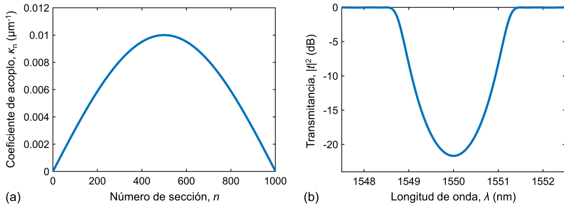
Figura 2.16. Simulación de un filtro con apodización sinusoidal mediante el TMM: (a) perfil de coeficiente de acoplo y (b) respuesta en transmitancia obtenida. La apodización del filtro se realiza periodo a periodo, es decir, cada sección del filtro comprende un único periodo Bragg ( L_n = \Lambda_n ). Además, todos los periodos tienen la misma longitud ( \Lambda_n = 500 nm). Por simplicidad, se ha considerado que el coeficiente de autoacoplo es nulo en todos los periodos ( \kappa'_n = 0 ), de forma que todos los periodos Bragg están sintonizados a la misma longitud de onda Bragg, en este caso, \lambda_0 = 1550 nm (el índice efectivo de la guía sin perturbar es n_{\text{eff}}(\lambda_0) = 1.55 ). El filtro contiene un total de 1000 periodos, lo que equivale a una longitud total de 500 \mu\text{m} . El índice de grupo de la guía sin perturbar es n_{g,u}(\lambda_0) = 3.5 .
