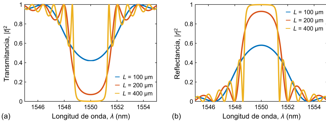
Figura 2.9. (a) Transmitancia y (b) reflectancia de un filtro Bragg no apodizado para diferentes longitudes de filtro: L = 100 \mu\text{m} (azul), L = 200 \mu\text{m} (rojo), y L = 400 \mu\text{m} (amarillo). Parámetros fijos en todas las curvas: \lambda_0 = 1550 nm, n_{g,u}(\lambda_0) = 3.5 , y \kappa = 0.01 \mu\text{m}^{-1} .
