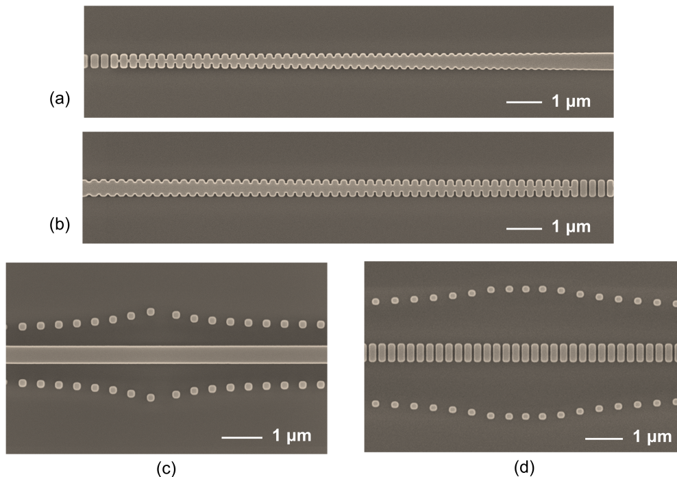
Figura 3.22. Imágenes SEM de algunas de las estructuras fabricadas: (a) transición de acoplador fibra-chip a guía de interconexión de entrada; (b) taper de guía Si-wire a guía SWG; (c) sección del filtro astrofotónico con núcleo Si-wire y para polarización TM; (d) sección del filtro astrofotónico con núcleo SWG y para polarización TM. Estas imágenes fueron tomadas antes la deposición del cladding superior.
