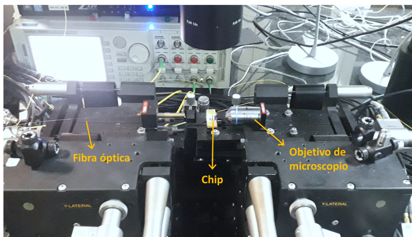
Figura 3.24. Foto del montaje de medida usado para caracterizar las estructuras fabricadas. A la izquierda y la derecha se muestran, respectivamente, las etapas de nanoposicionamiento de la fibra óptica a la entrada y del objetivo de microscopio a la salida. En el centro se coloca el chip fotónico a caracterizar.
