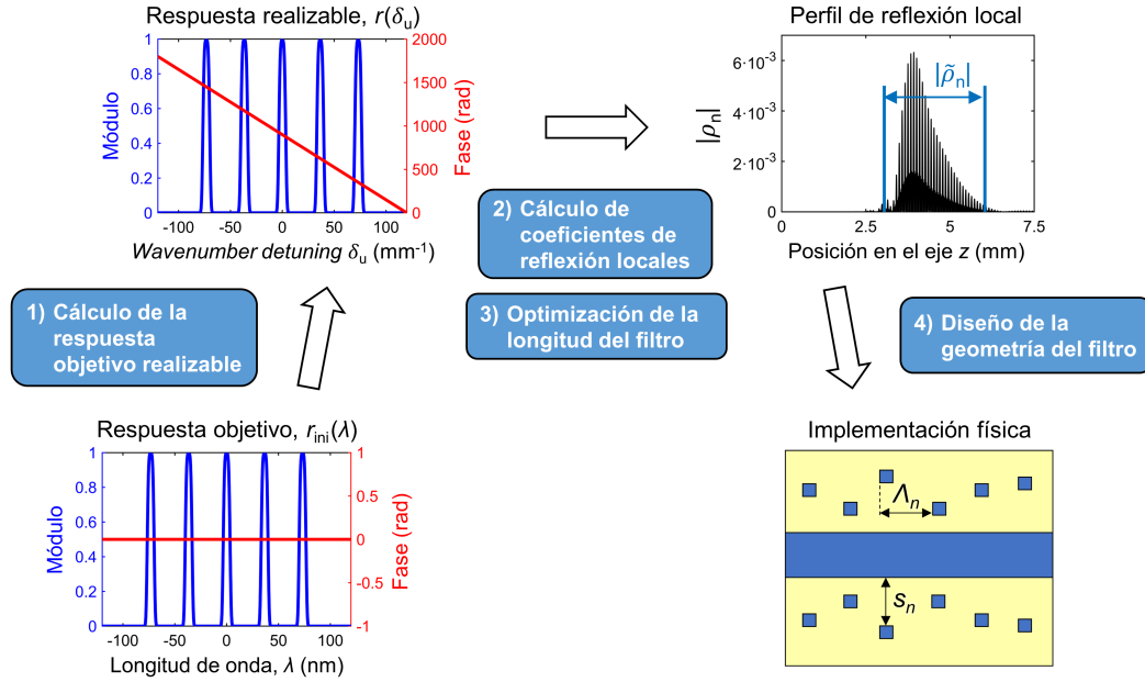
Figura 2.18. Representación gráfica del procedimiento de diseño de filtros Bragg apodizados de respuesta espectral arbitraria que se propone en esta tesis, basado en los algoritmos LP y LA. Como ejemplo, se muestra el diseño de un filtro objetivo con cinco bandas de reflexión a longitudes de onda arbitrarias.
