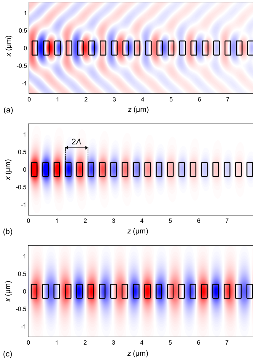
Figura 2.3. Propagación de campo eléctrico (polarización TE) del modo Floquet-Bloch de una estructura periódica funcionando en (a) régimen de radiación, (b) régimen de Bragg, y (c) régimen sub longitud de onda. Resultados obtenidos mediante simulación electromagnética 2D, utilizando un software de simulación interno [65]. Datos de la estructura: la longitud del periodo es 400 nm; los segmentos que forman la guía periódica tienen anchura 400 nm y longitud 200 nm; el índice de refracción de los segmentos es 2.2 y el del sustrato 1.5. Longitud de onda de trabajo: (a) \lambda = 1.04 \mu\text{m} , (b) \lambda = 1.47 \mu\text{m} , y (c) \lambda = 1.65 \mu\text{m} .
