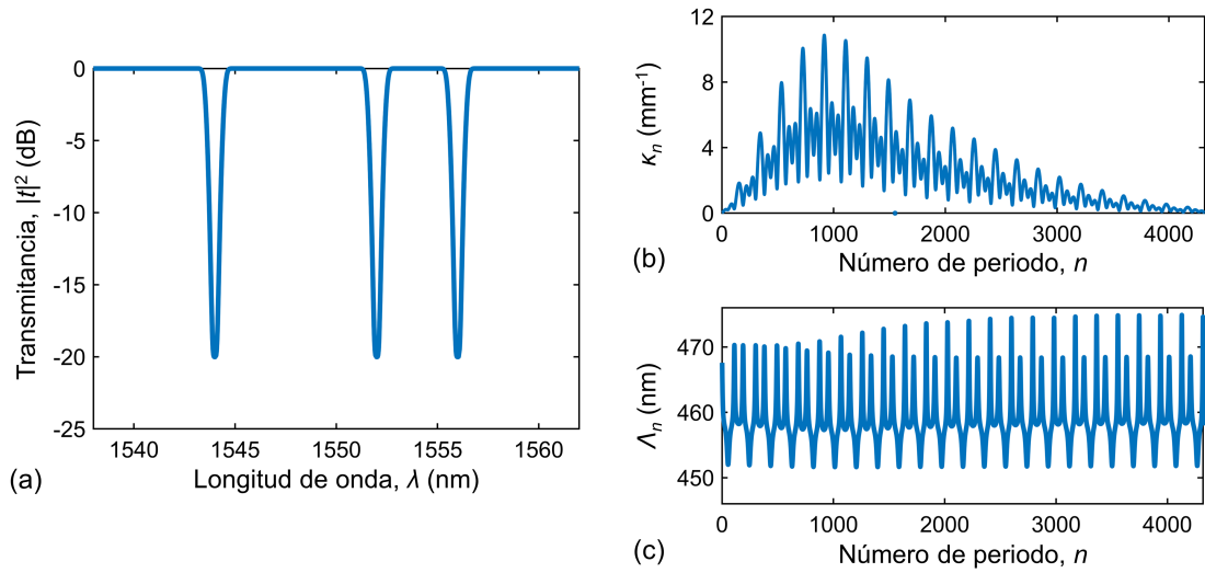
Figura 4.8. Diseño nominal del filtro de tres notches utilizado para comparar los modelos de ruido de fase discreto y continuo: (a) transmitancia espectral sintetizada, obtenida mediante el TMM; (b) perfil de coeficiente de acoplo; (c) perfil de periodo Bragg.
