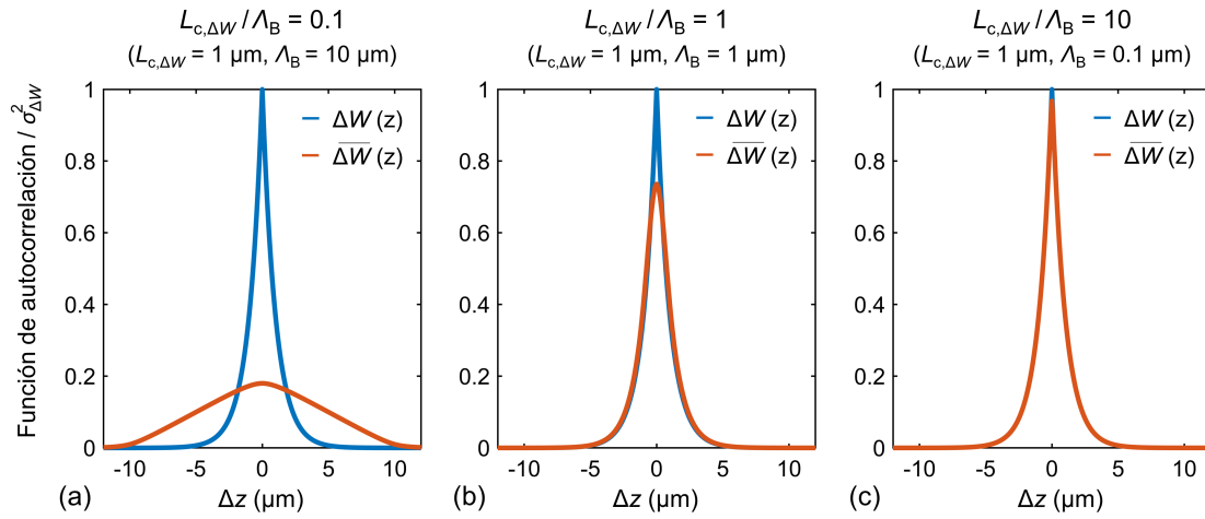
Figura 4.4. Función de autocorrelación del error de anchura continuo, \Delta W (azul), y del error de anchura promedio en cada periodo, \overline{\Delta W}(z) (rojo), en función de la distancia espacial \Delta z , ambas normalizadas por la varianza del proceso original \sigma_{\Delta W}^2 . Se ilustran tres casos: (a) L_{c,\Delta W}/\Lambda_B = 0.1 , (b) L_{c,\Delta W}/\Lambda_B = 1 , y (c) L_{c,\Delta W}/\Lambda_B = 10 . En todas las gráficas se ha mantenido la misma longitud de correlación, L_{c,\Delta W} = 1 \mu\text{m} , variándose la longitud del periodo Bragg \Lambda_B .
