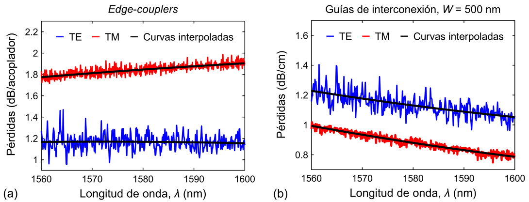
Figura 3.27. Estimación de (a) pérdidas de los edge-couplers y (b) pérdidas de propagación de las guías de interconexión con respecto a la longitud de onda \lambda . En azul y rojo se muestran los resultados obtenidos para polarización TE y TM, respectivamente, habiendo aplicado el mismo procedimiento de cálculo que en la figura 3.26. En negro se representa el resultado de interpolar con una función cuadrática los resultados de las curvas azules y rojas. Las curvas negras son las que se utilizarán para descontar el efecto de las pérdidas de los edge-couplers y las guías de interconexión en las medidas de los filtros.
