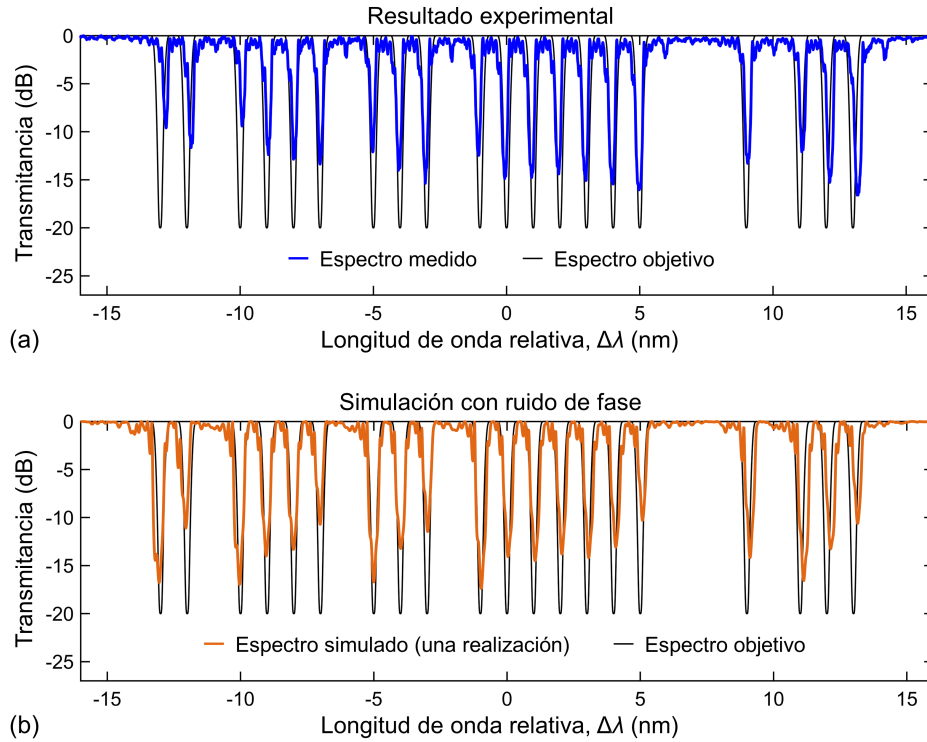
Figura 4.10. Comparación de espectro medido y espectro simulado con ruido de fase para el filtro astrofónico con núcleo Si-wire y polarización TM: (a) respuesta medida (azul) y respuesta objetivo (negro); (b) respuesta simulada para una realización aleatoria de ruido de fase (naranja) y respuesta objetivo (negro). Se han utilizado los siguientes parámetros para definir el ruido de fase: \sigma_{\Delta W} = 2 nm y L_{c,\Delta W} = 15 \mu m.
