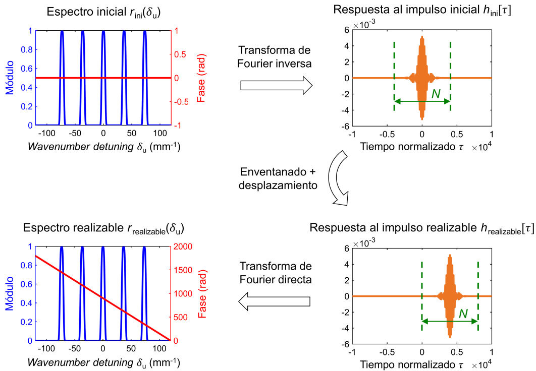
Figura 2.19. Representación gráfica del proceso aplicado sobre la respuesta espectral ideal para obtener una respuesta físicamente realizable. Este espectro realizable es el que se toma como objetivo para el resto del proceso de diseño.
