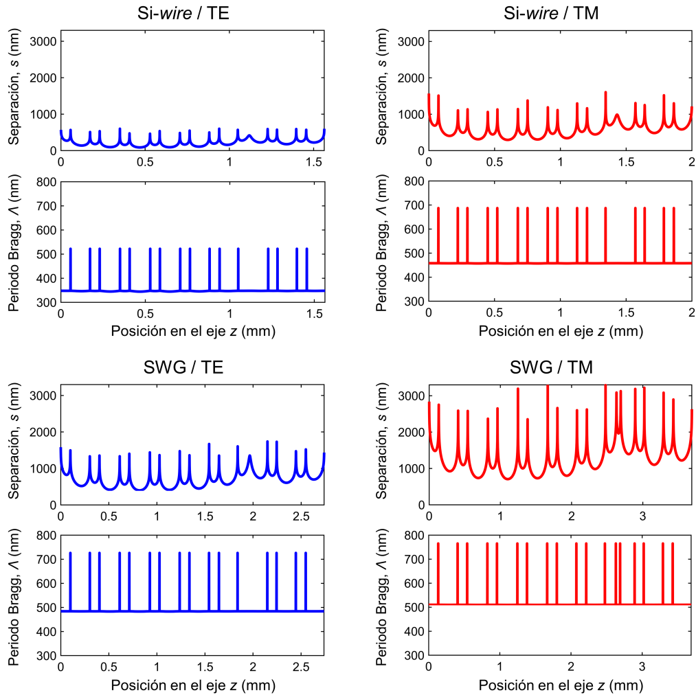
Figura 3.16. Perfiles de separación lateral y periodo Bragg de filtros flat-top multicanal para las diferentes configuraciones de filtro. Los resultados corresponden a un filtro flat-top de tres canales con los siguientes parámetros objetivo: r_{\max} = 0.995 , \Delta\lambda_{3\text{dB}} = 0.8 \text{ nm} y \Delta\lambda_{\text{canal}} = 1.6 \text{ nm} .
